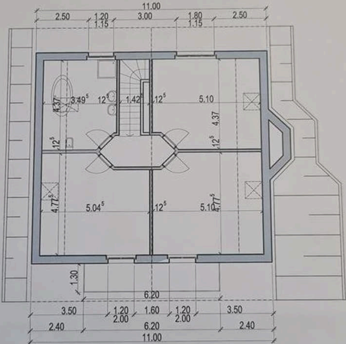
Grundriss DG
