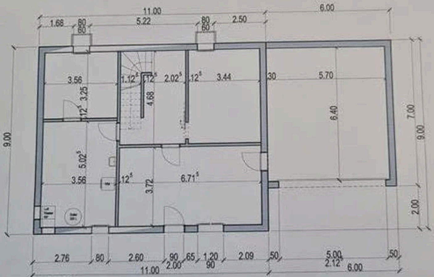
Grundriss UG
