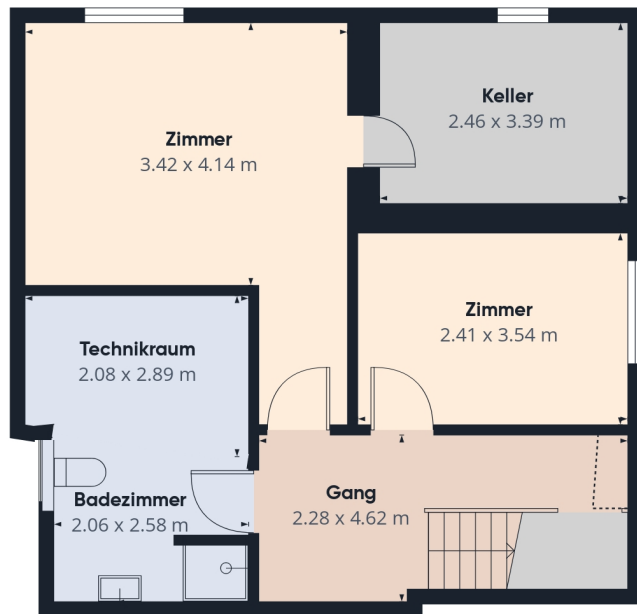
Etage -1
