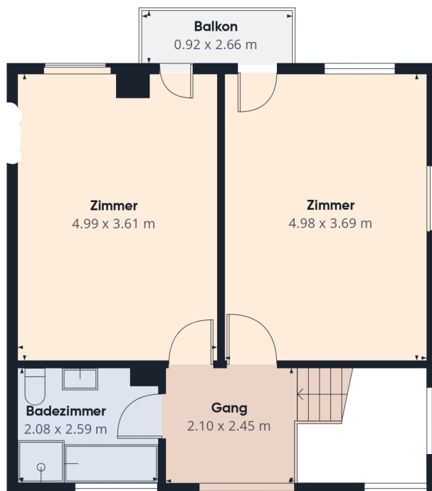
Etage 1
