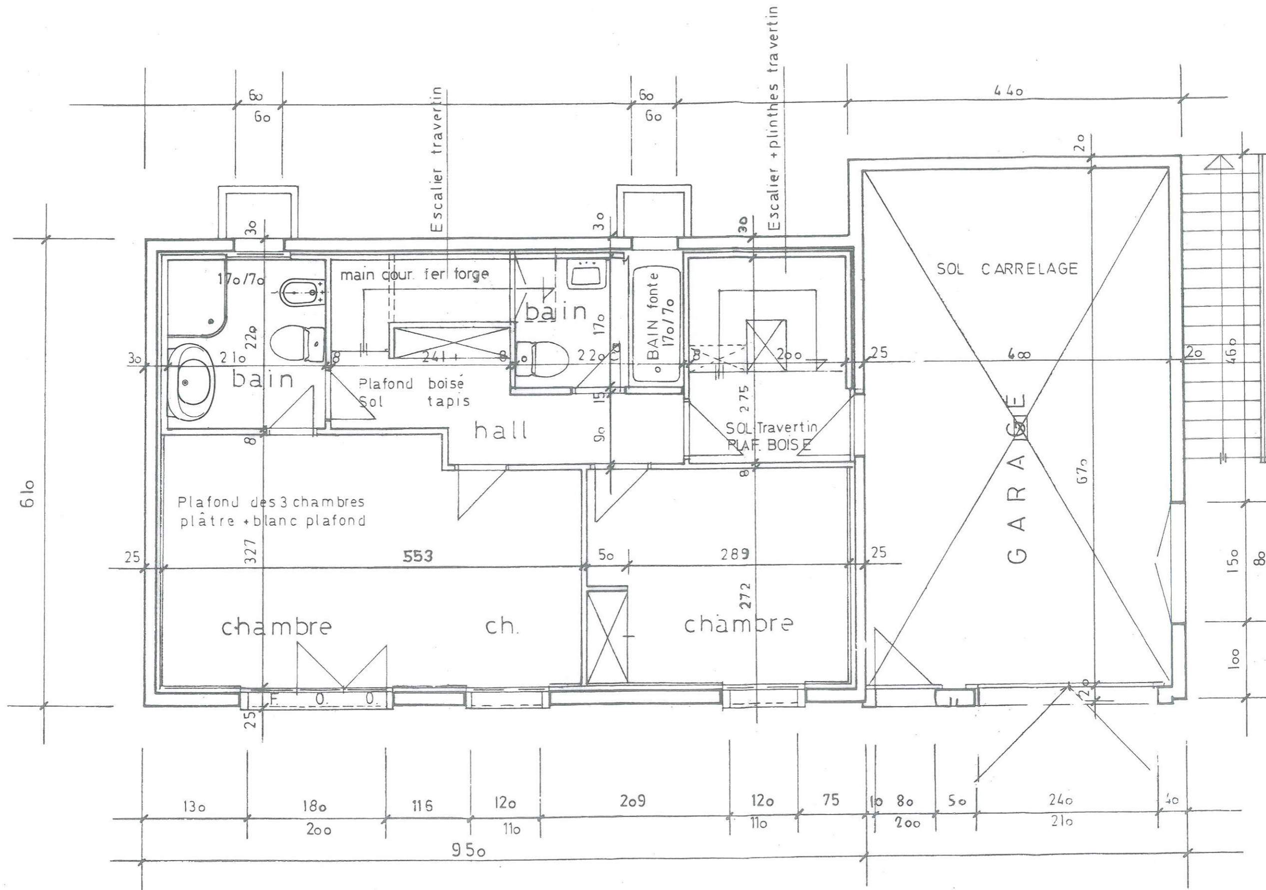
REZ - DE - CHAUSSEE
