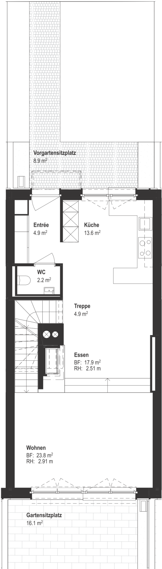
Erdgeschoss
