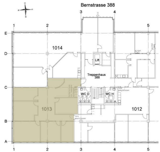
Grundriss 191 m2
