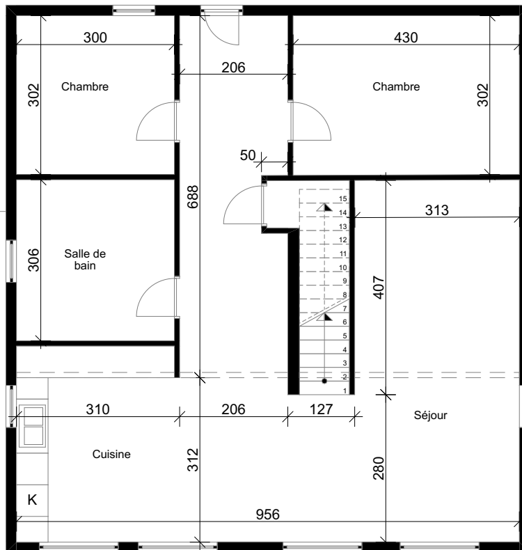
Rez-de-Chaussée
