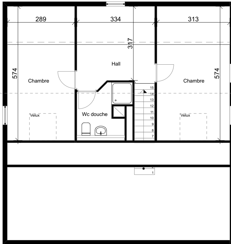
Etage 1
