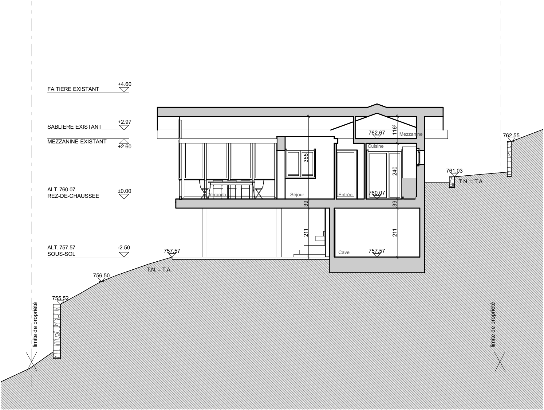
COUPE B
