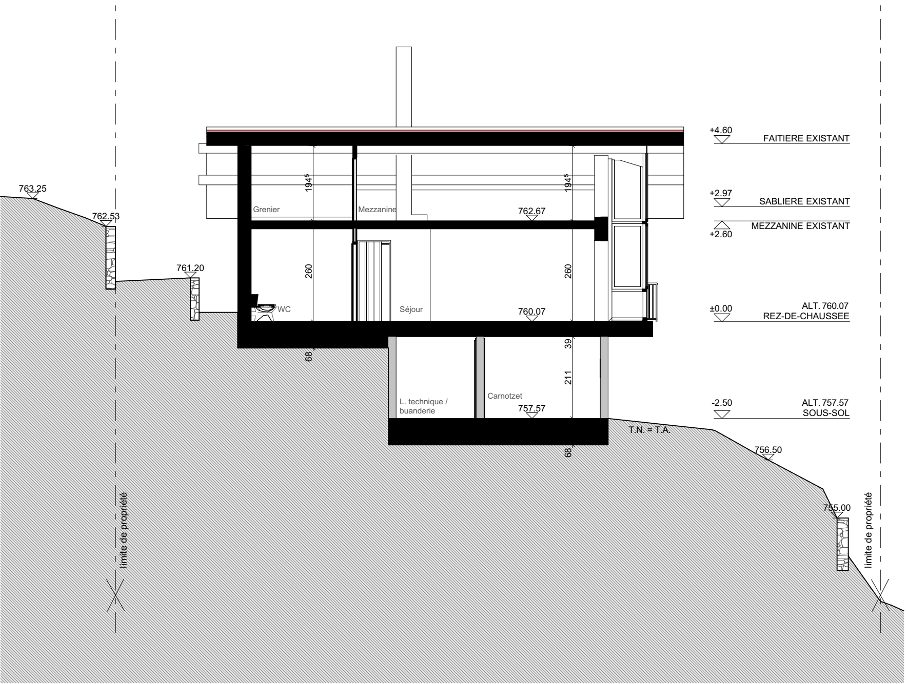
COUPE C
