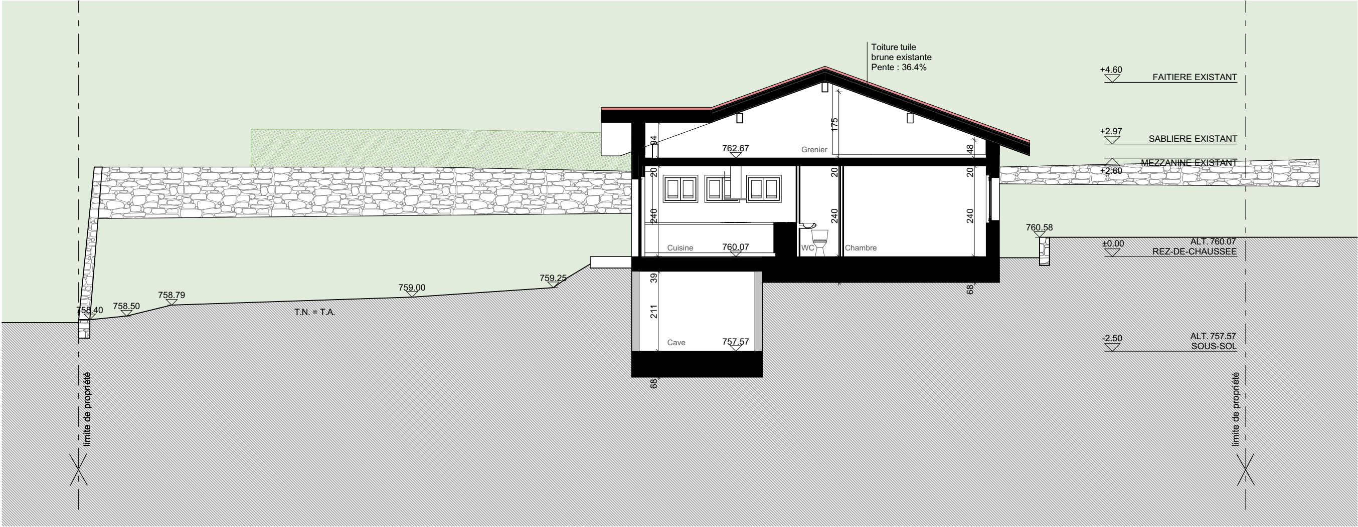
COUPE A
