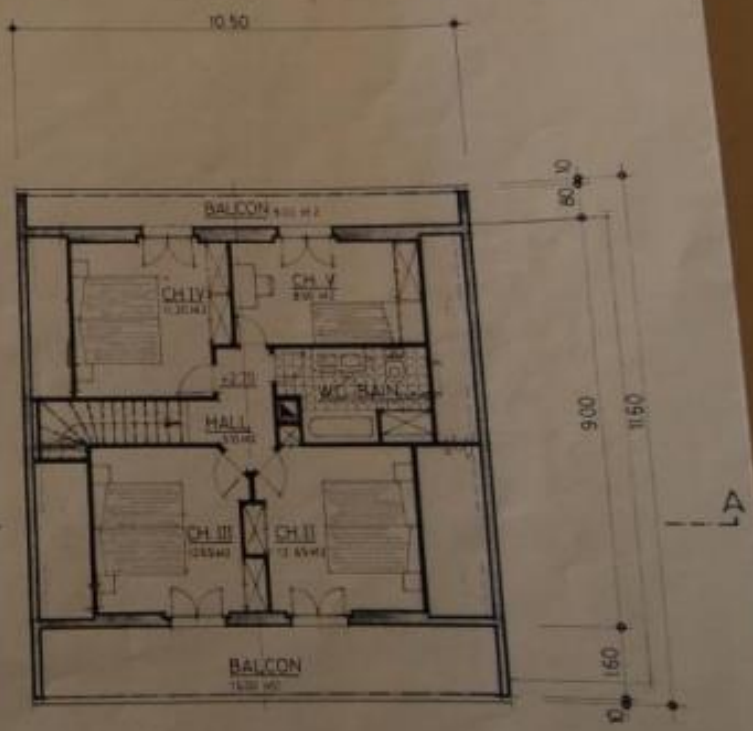
ETAGE 1:100
