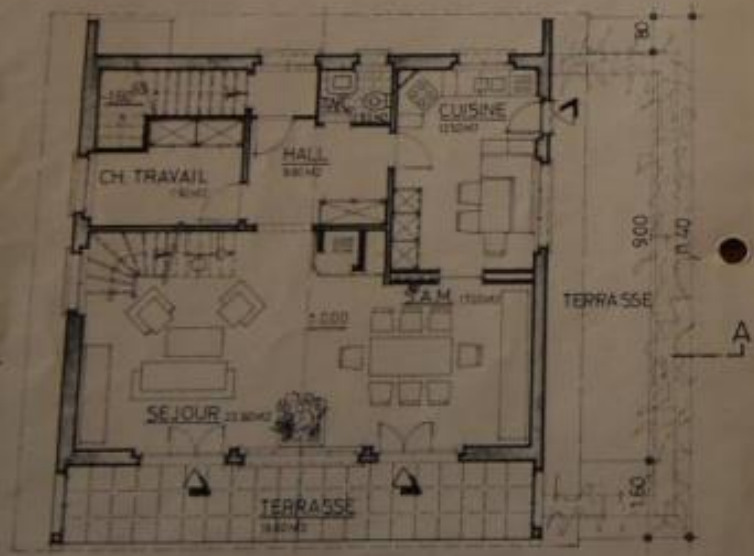
REZ DE CHAUSSEE 1:100
