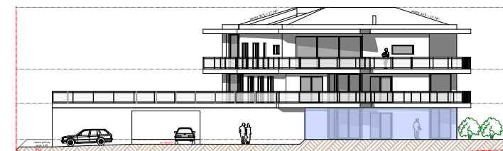
SUD-OUEST
