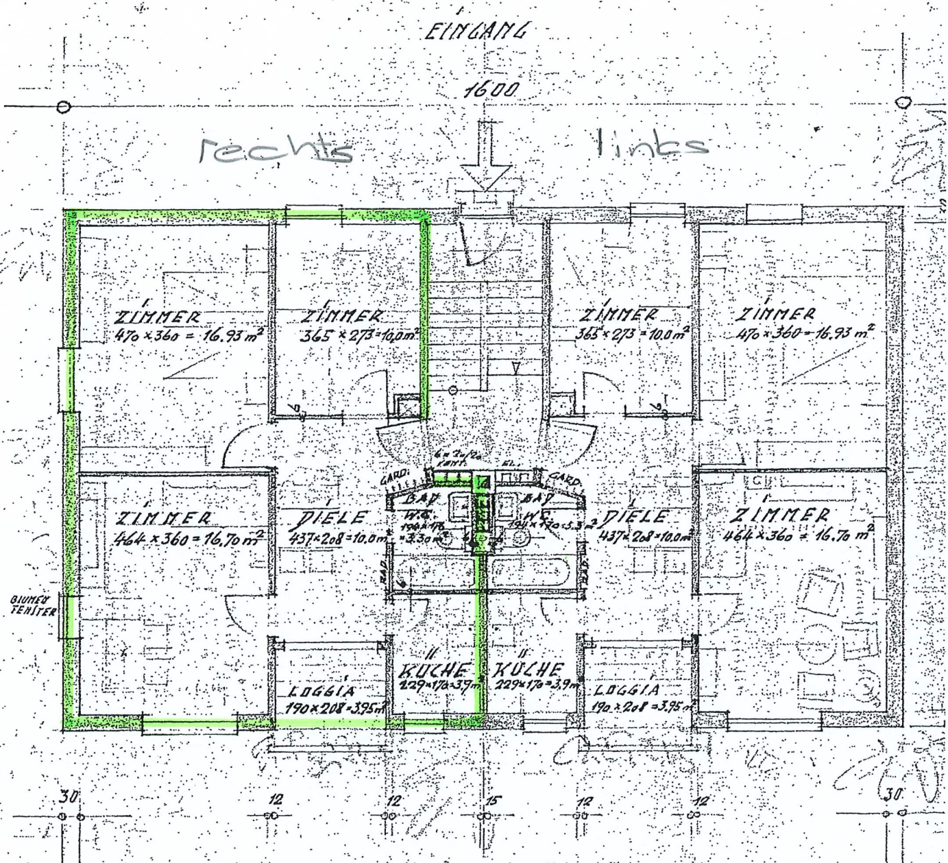
ERD- & OBERGESCHOSS
