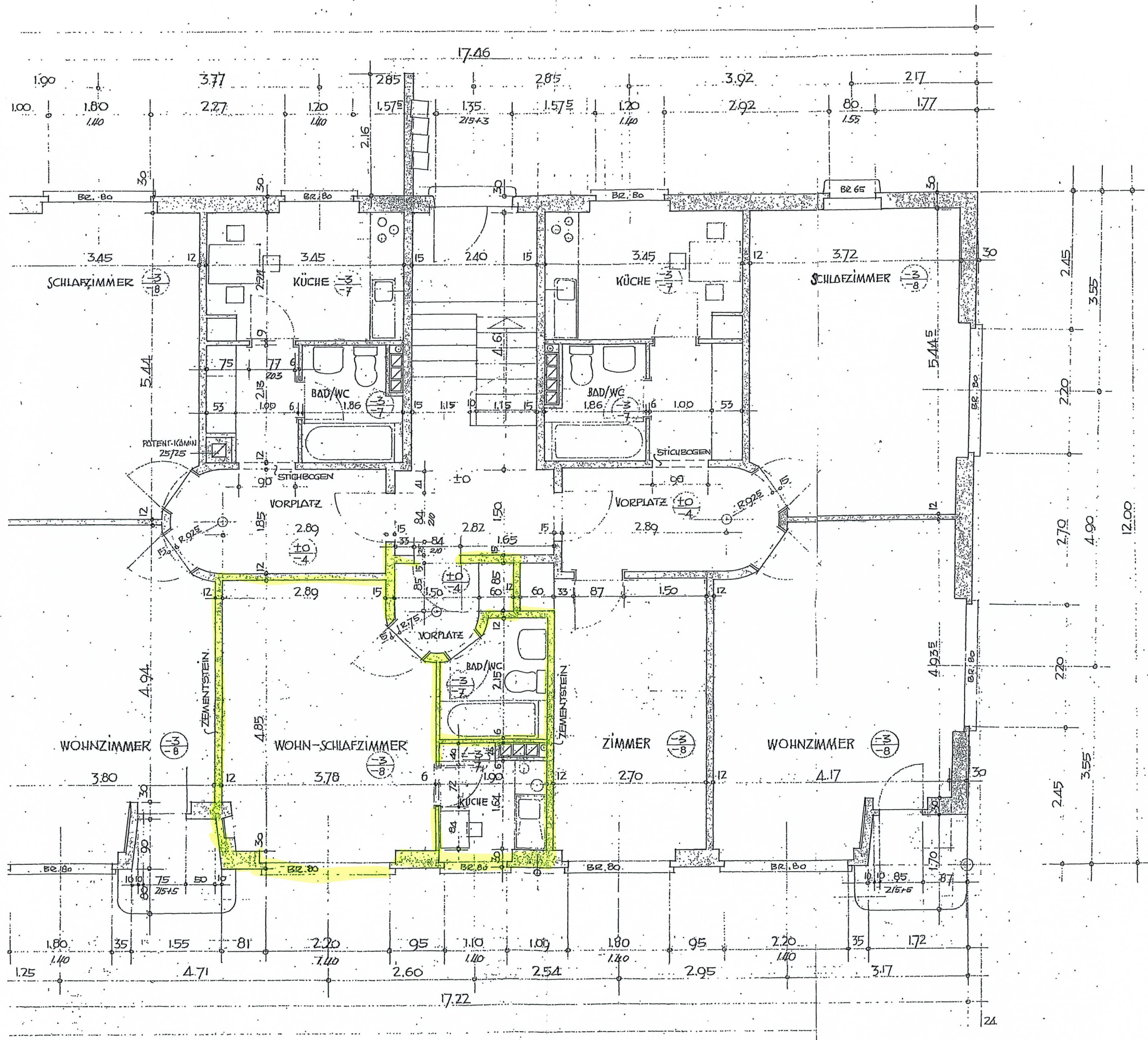
ROSENWEG 10 ERDGESCHOSS-GRUNDRISS M: 1:50
