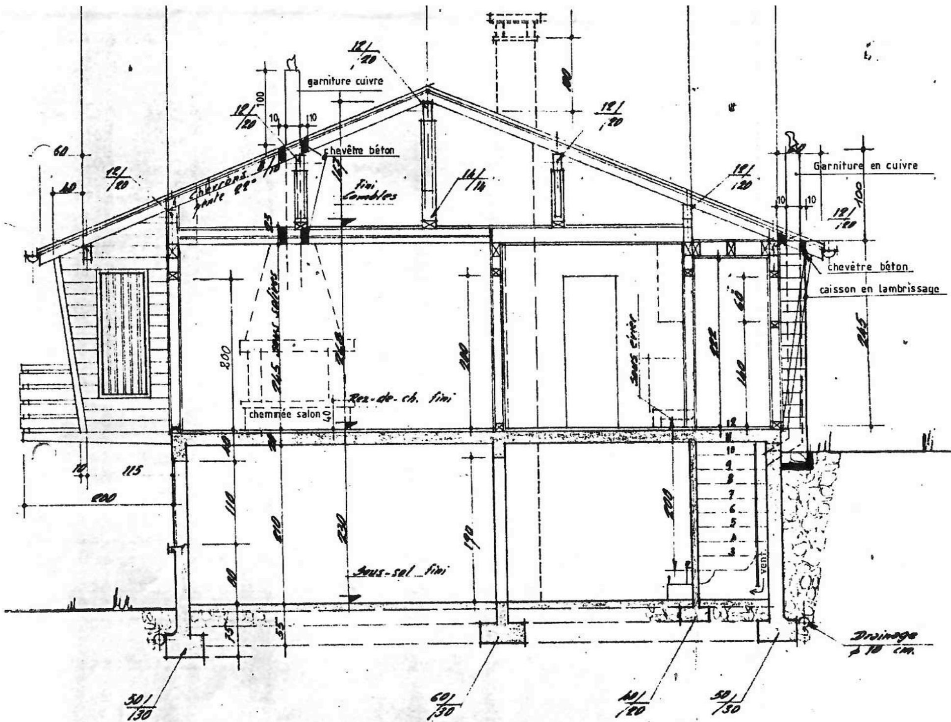
Coupe A-A
