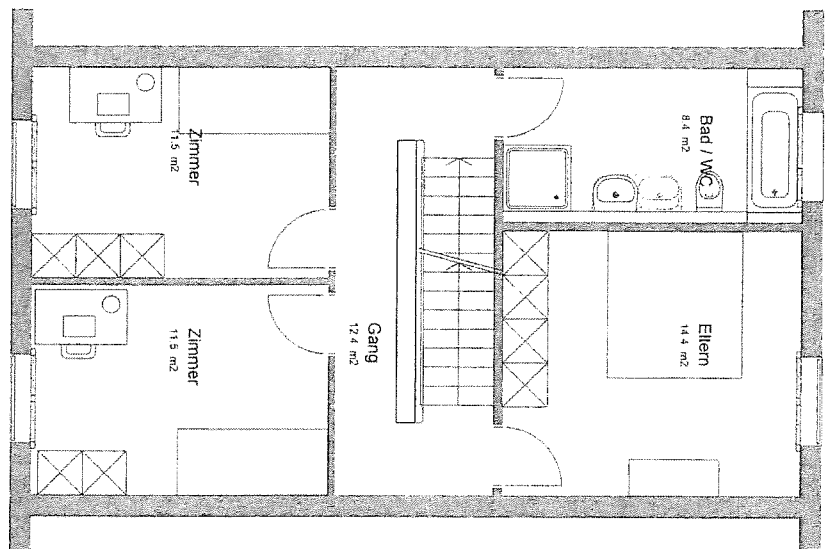
OBERGESCHOSS
