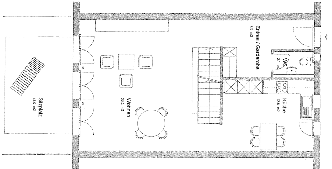
ERDGESCHOSS
