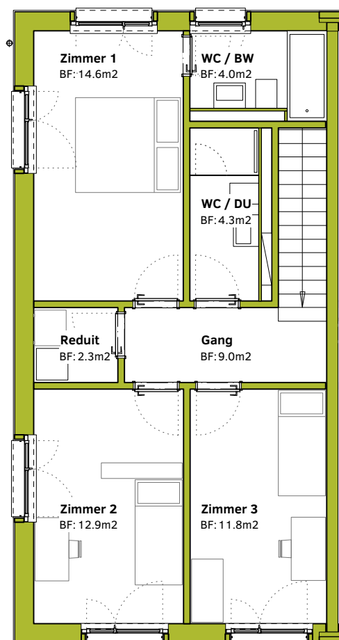
Obergeschoss
