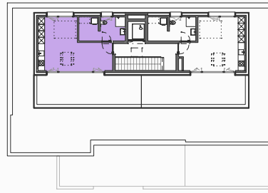
ÜBERSICHT ATTIKAGESCHOSS MST.: 1:500
