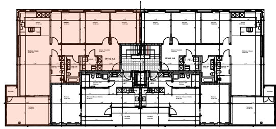
ÜBERSICHT 1. OBERGESCHOSS
