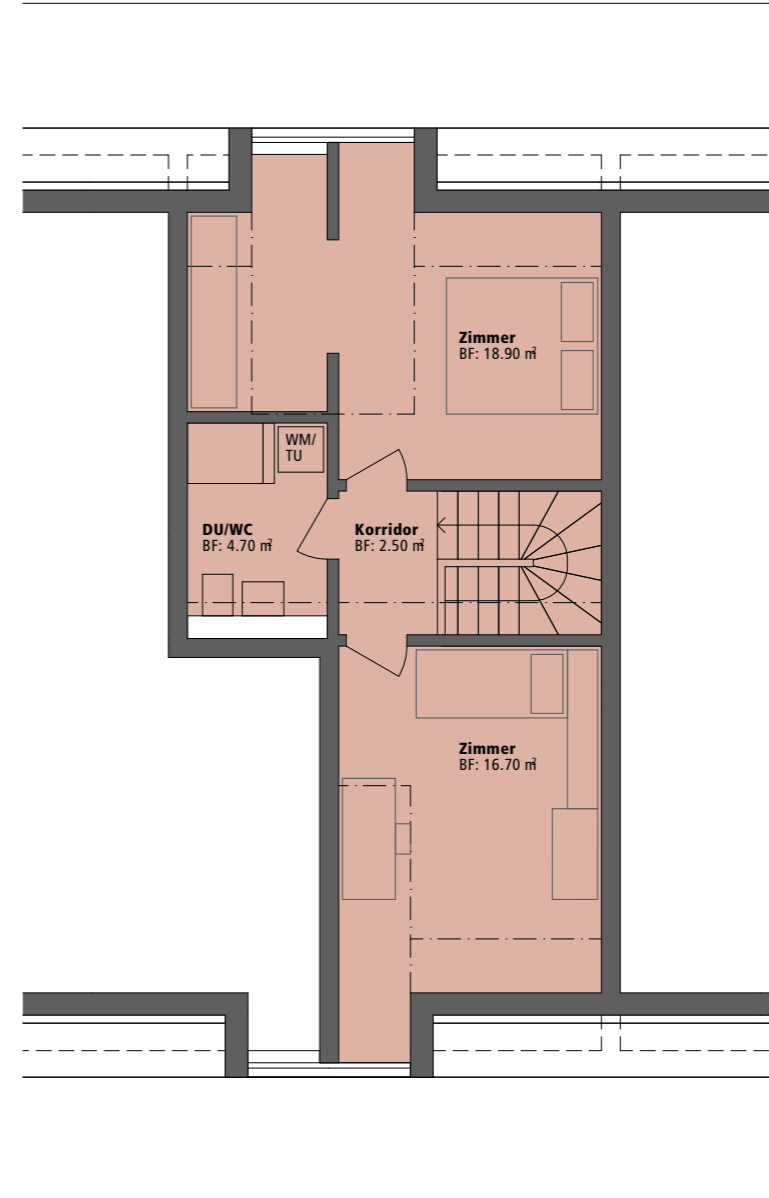
Dachgeschoss
