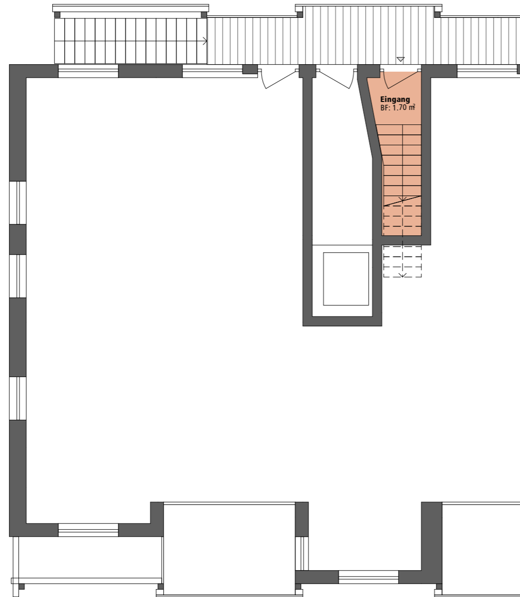
1. Obergeschoss Dazugehöriges Kellerabteil auf Übersichtsplan
