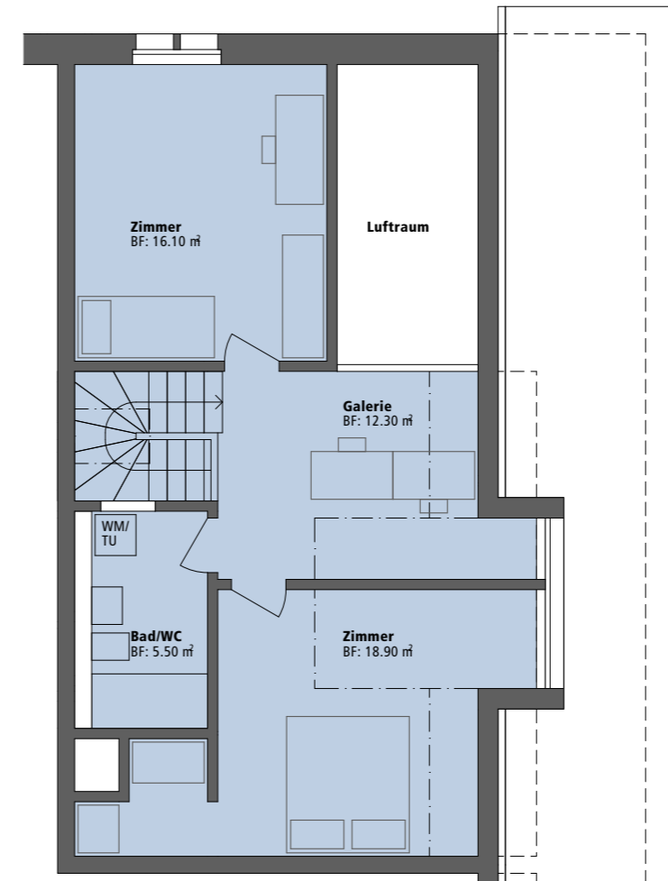
Dachgeschoss
