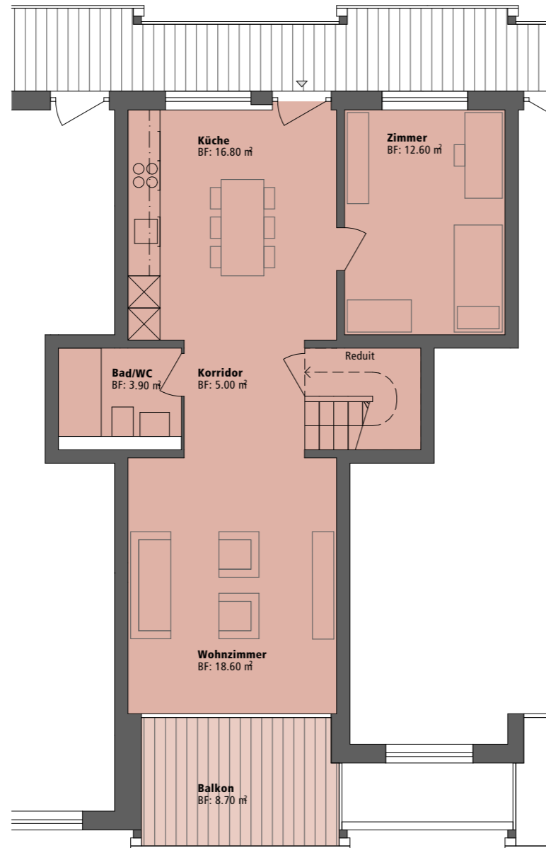
1. Obergeschoss Dazugehöriges Kellerabteil auf Übersichtsplan
