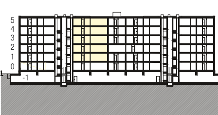
Sezione tipo
