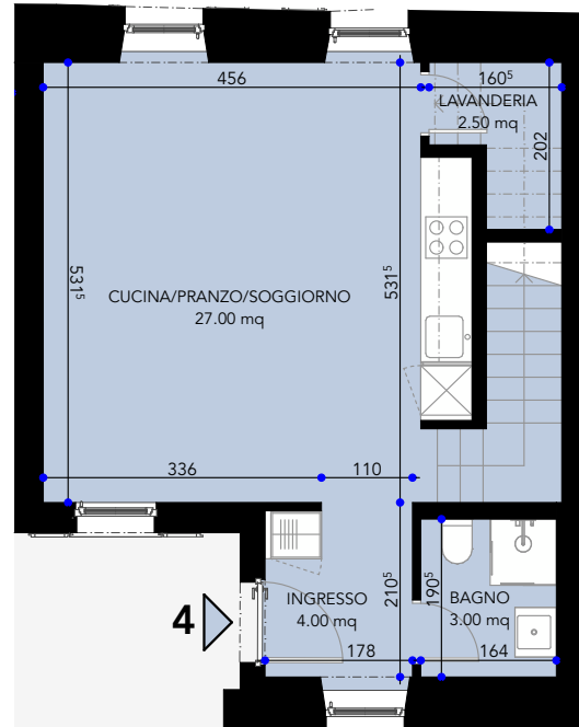
PIANO TERRA Altezza locali 3.19
