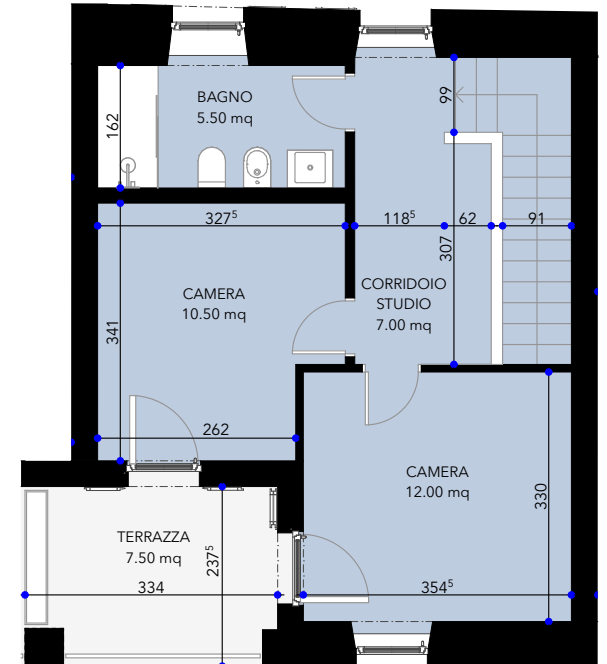
PIANO PRIMO Altezza locali da 3.20 a 4.30
