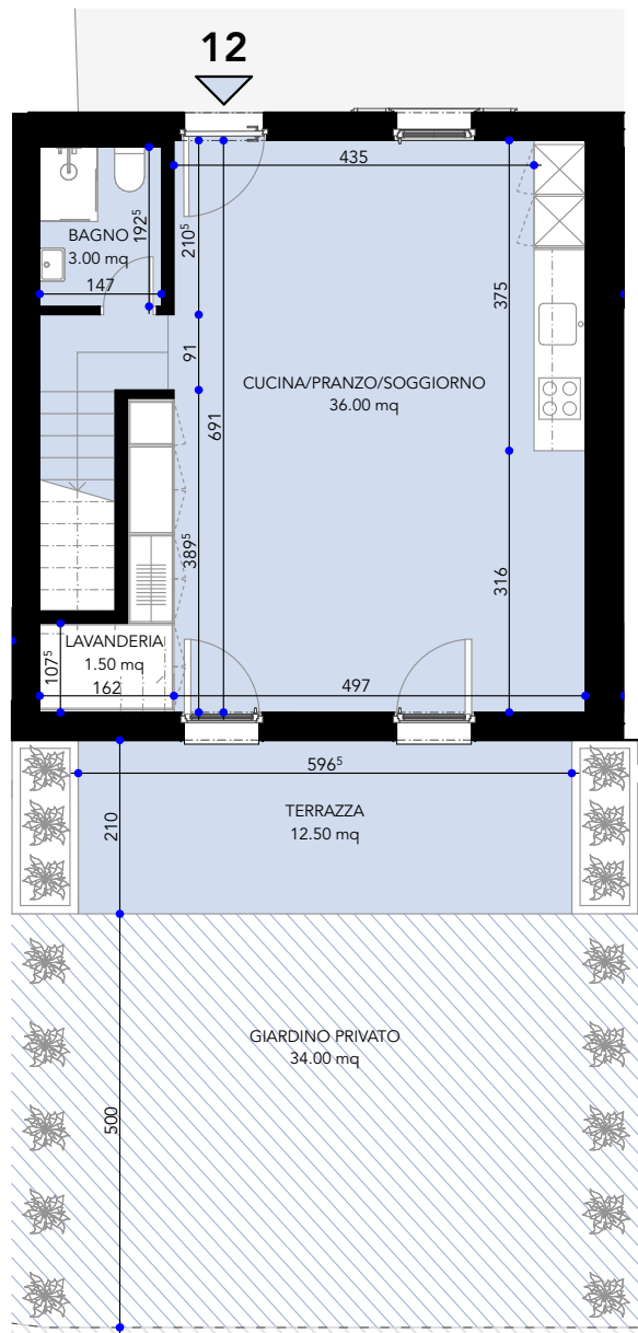
PIANO TERRA Altezza locali 2.64
