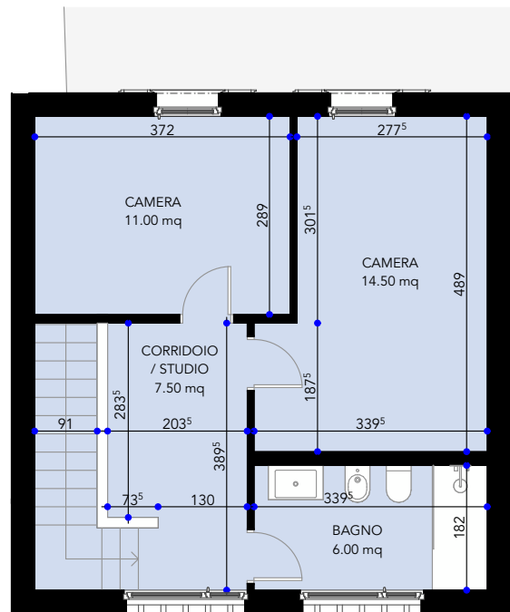
PIANO PRIMO Altezza locali da 2.60 a 3.60
