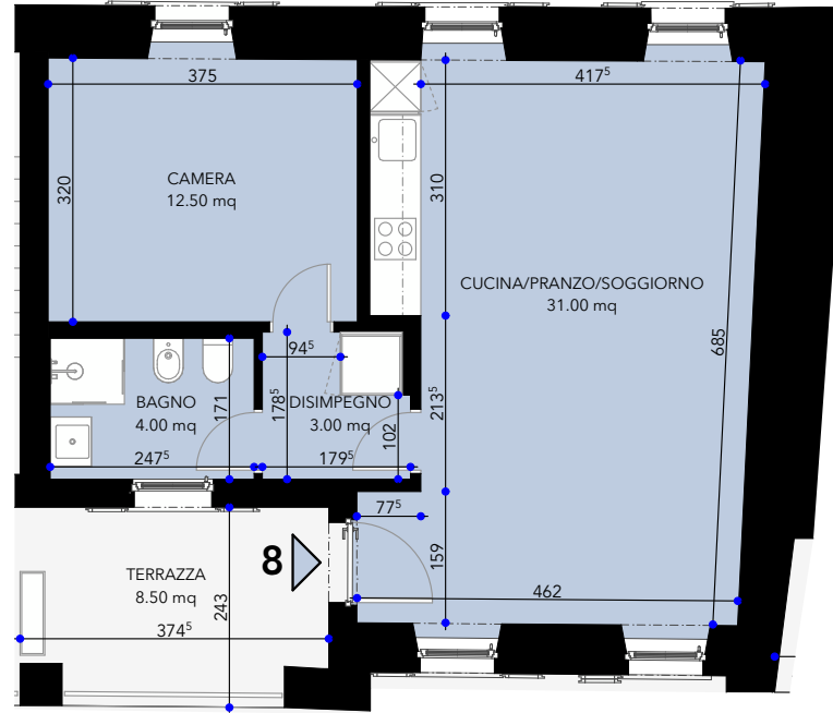
PIANO PRIMO Altezza locali 3.19
