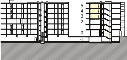
Sezione tipo
