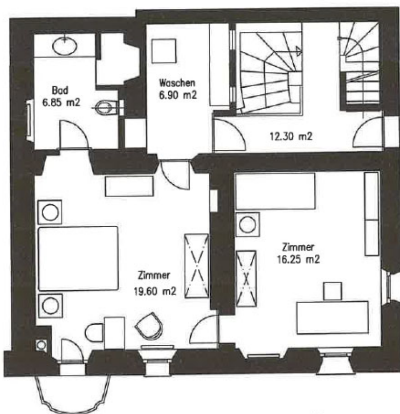
1. Obergeschoss Mst. 1:100
