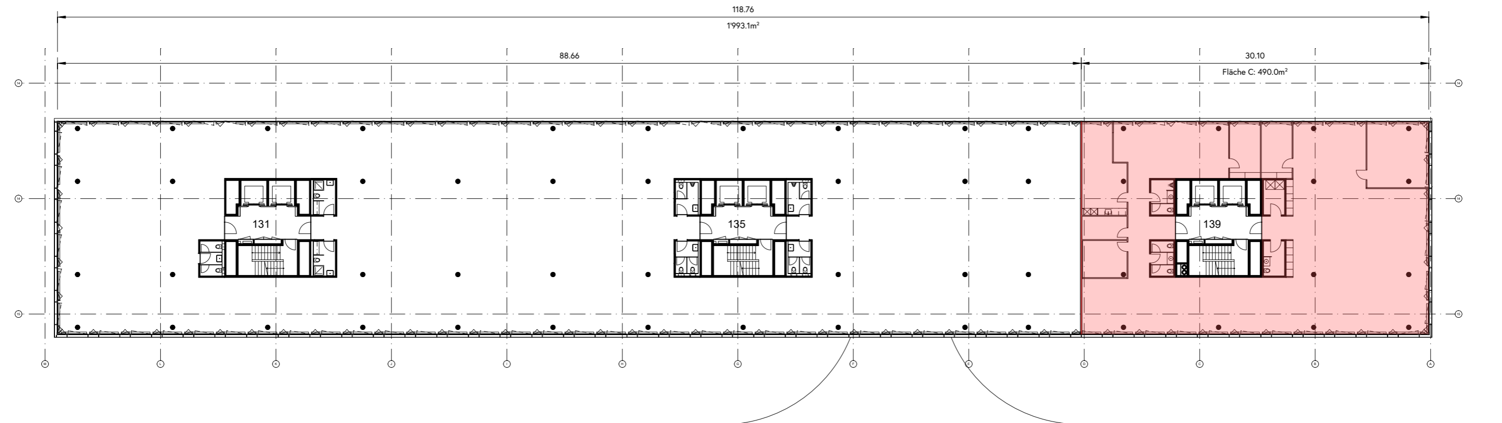
Grundriss 5.Obergeschoss 1:333
