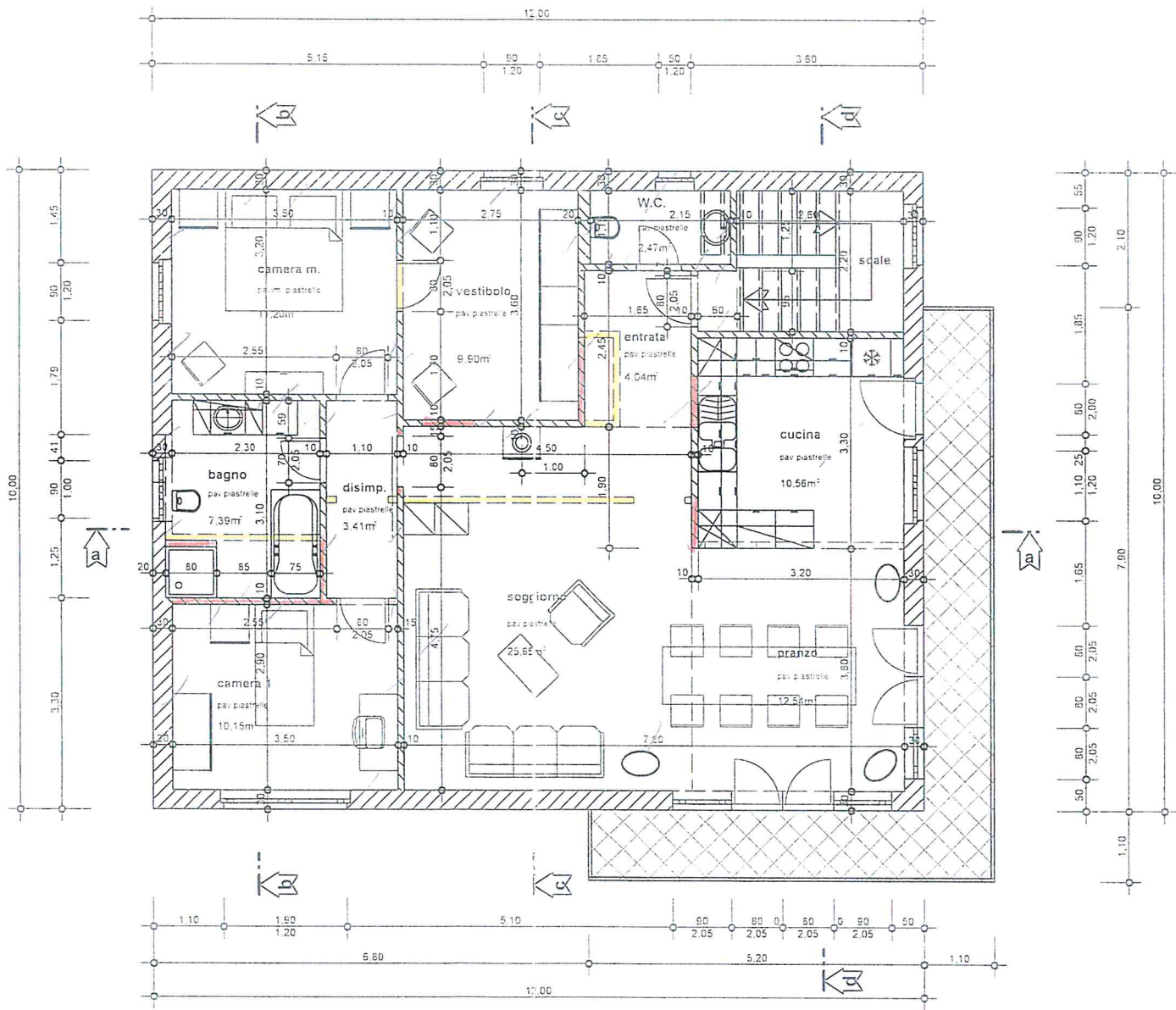
pianta piano abitabile
