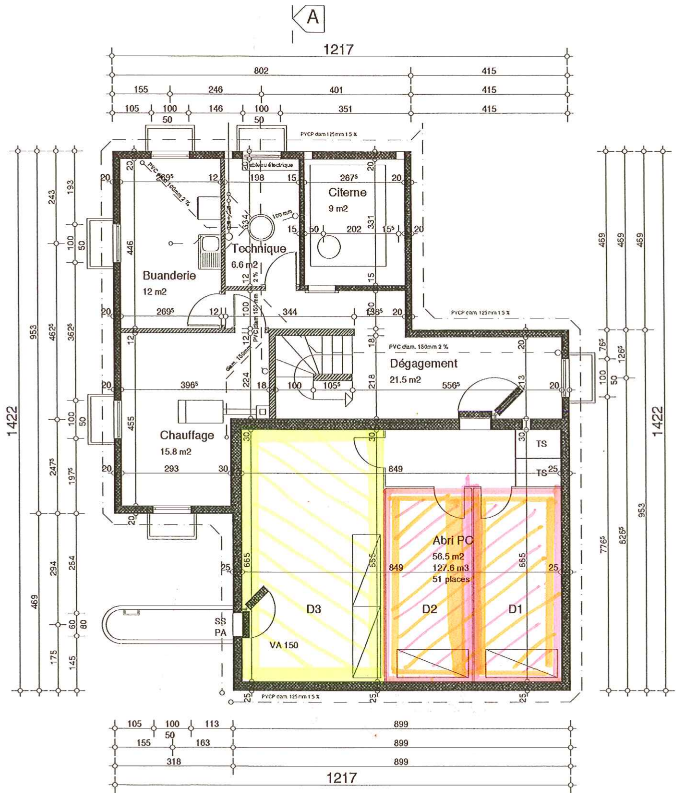
SOUS-SOL type "D"
