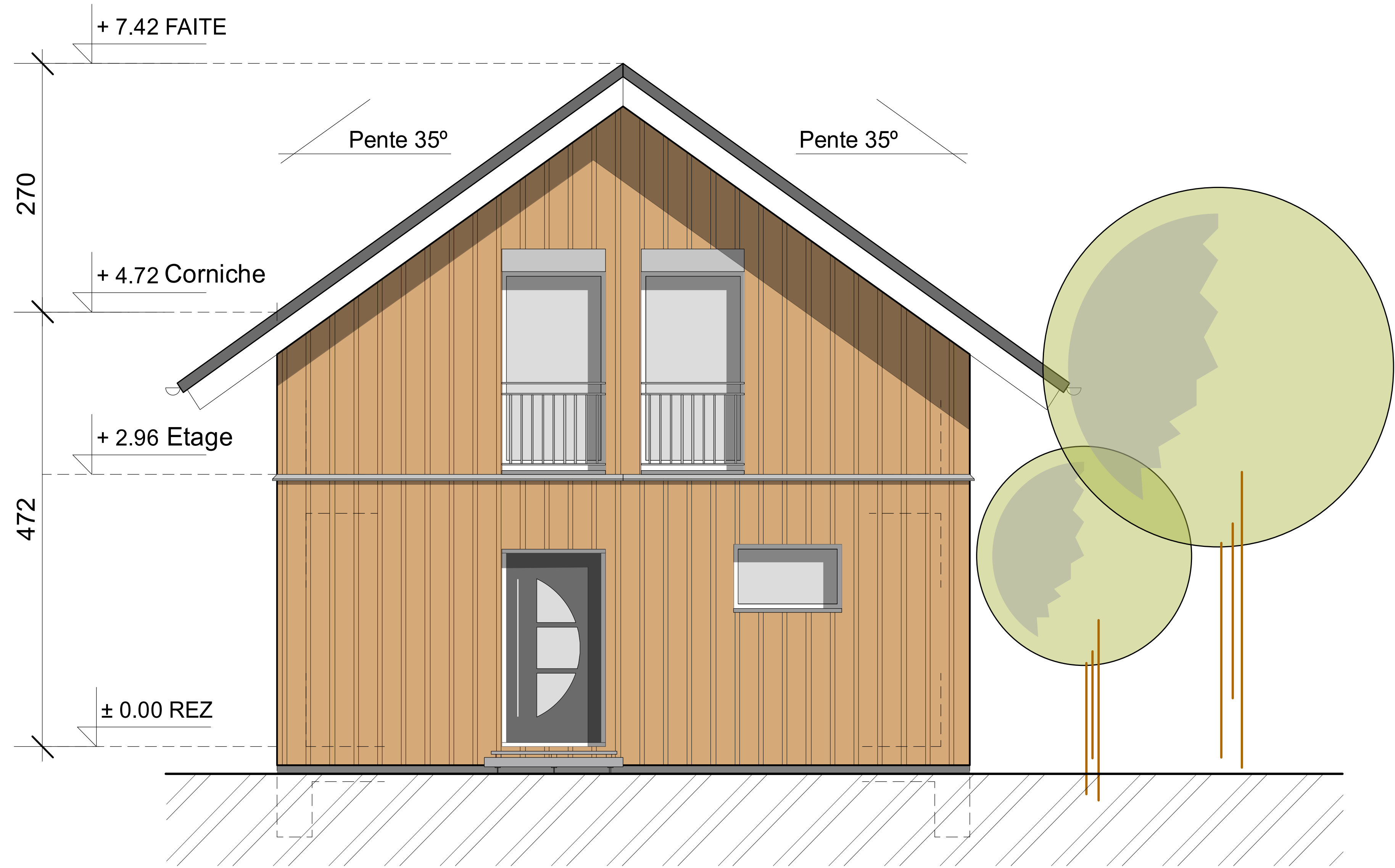
FACADE NORD
