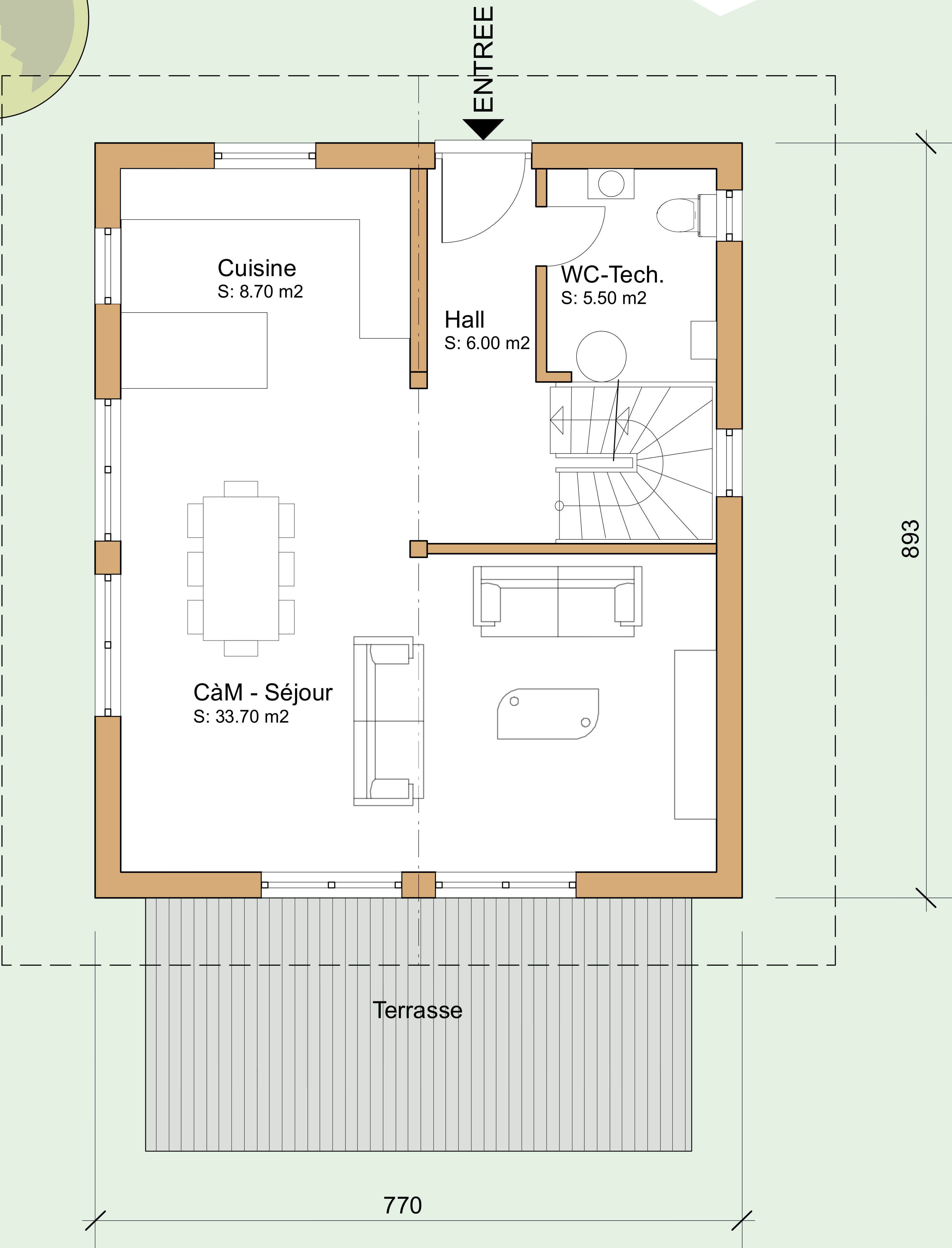
REZ-DE-CHAUSSEE
