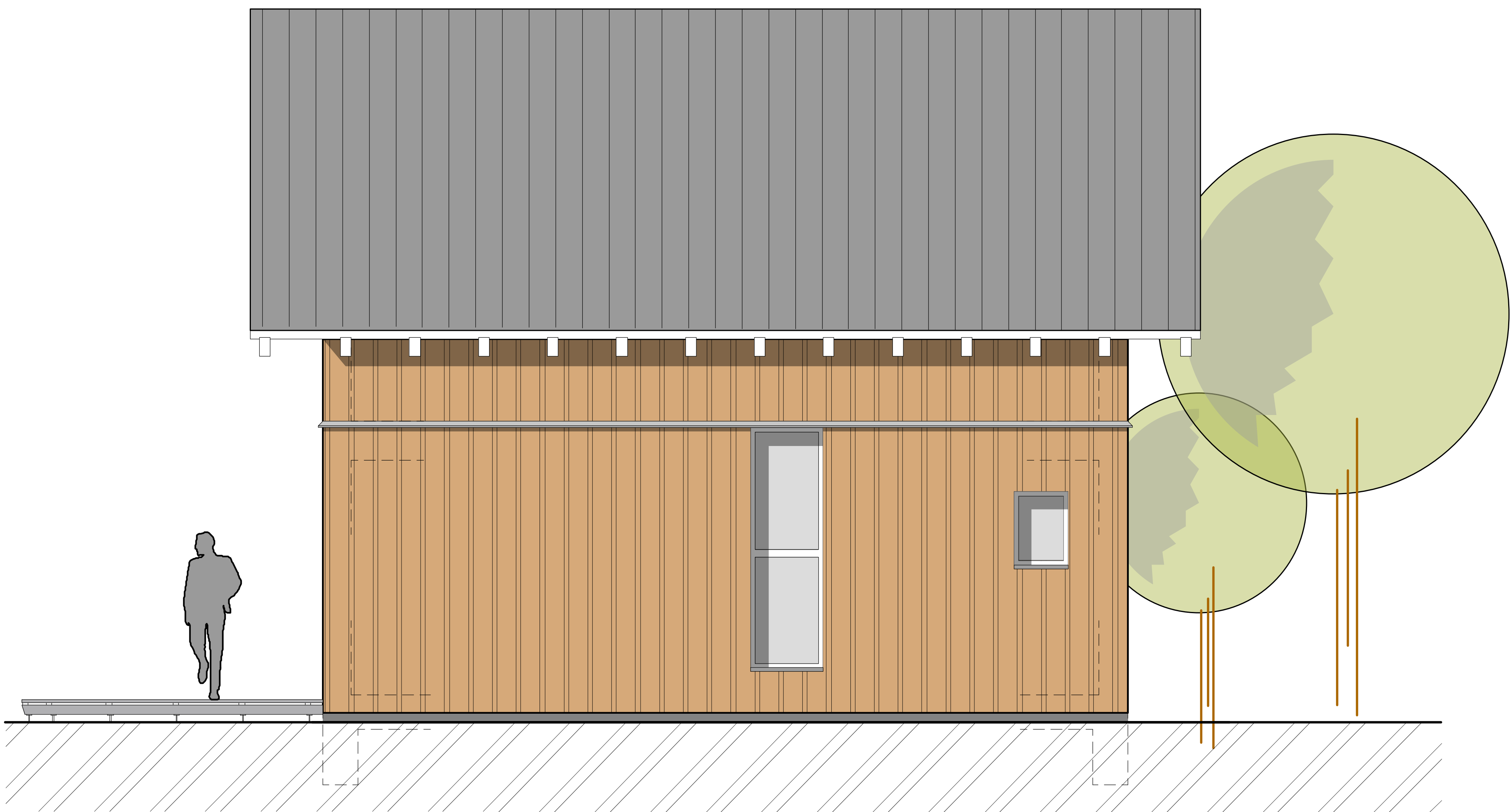
FACADE EST
