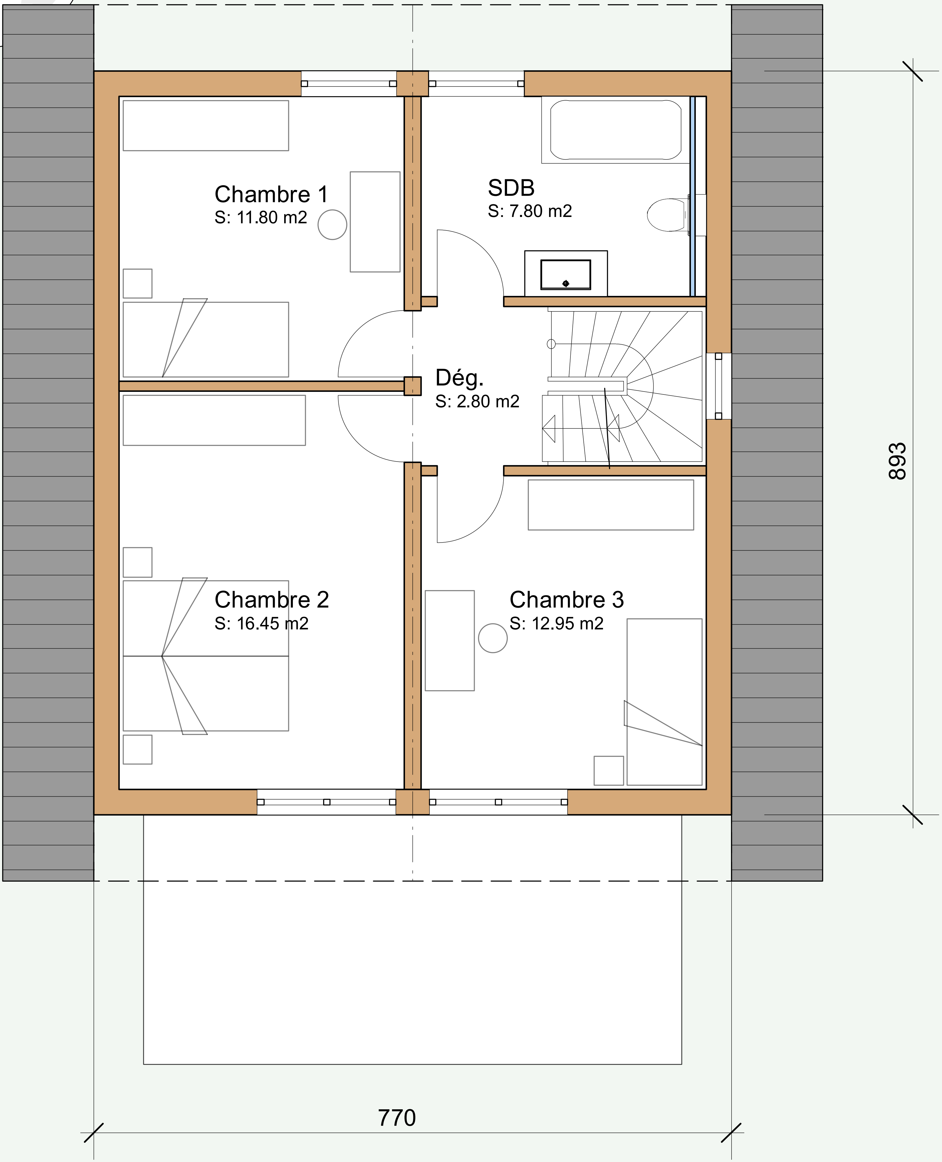
ETAGE
