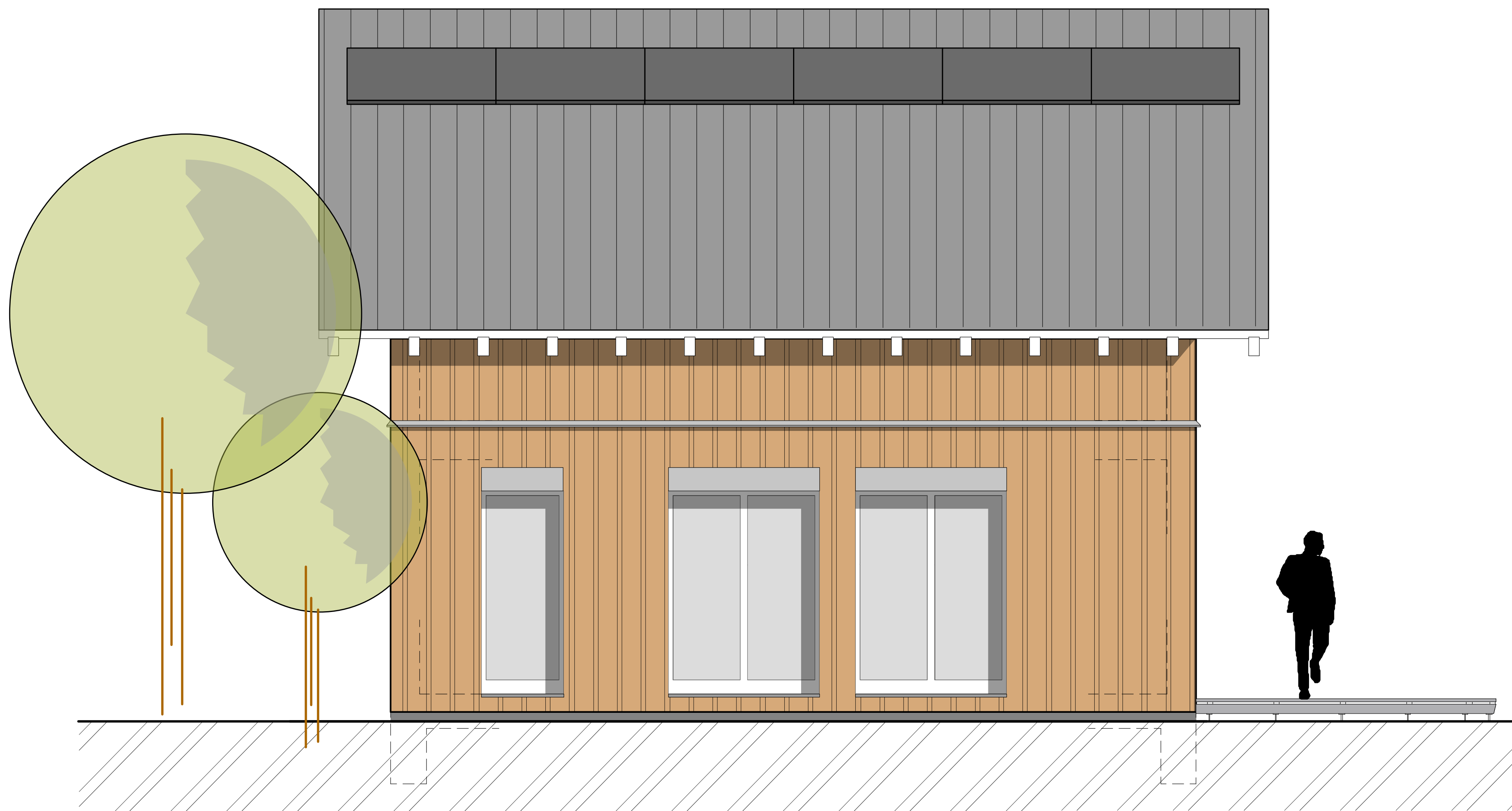
FACADE OUEST
