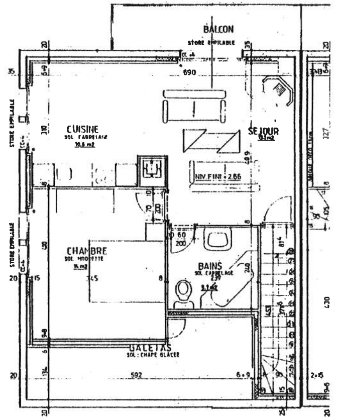
ÉTAGE
