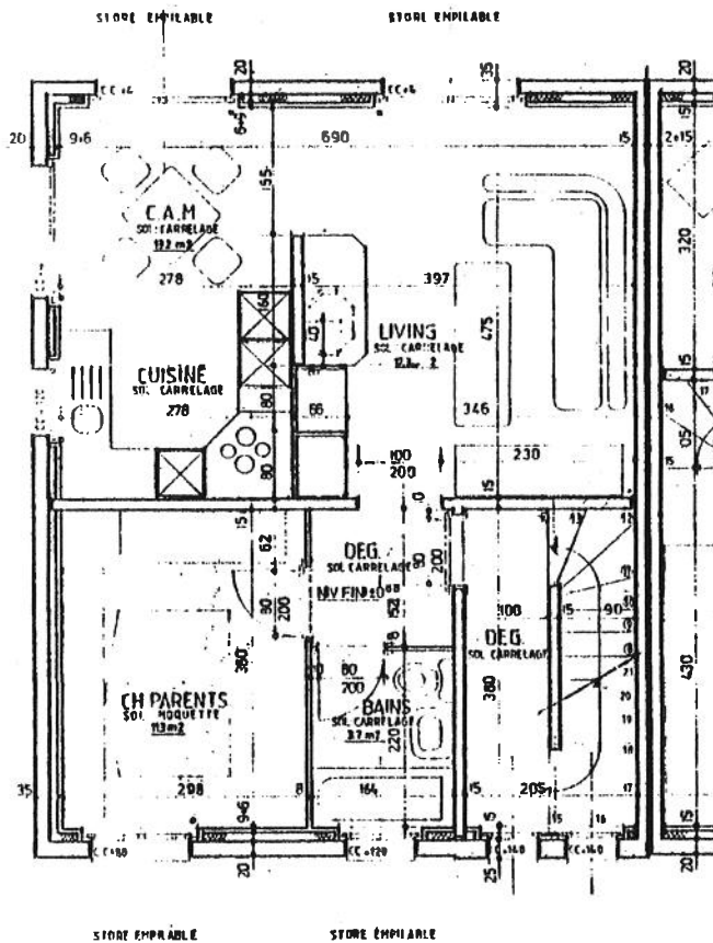
REZ-DE-CHAUSSÉE
