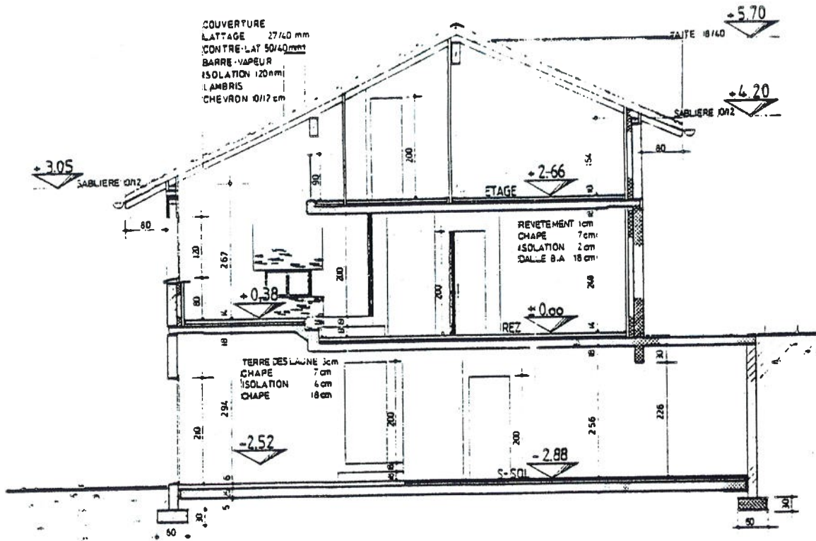
COUPE A-A
