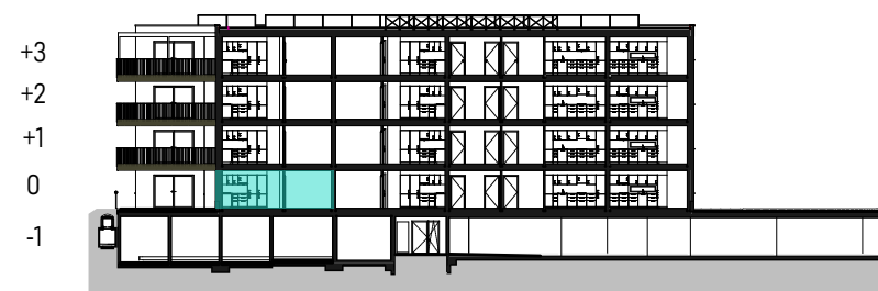
Coupe A-A 1/500
