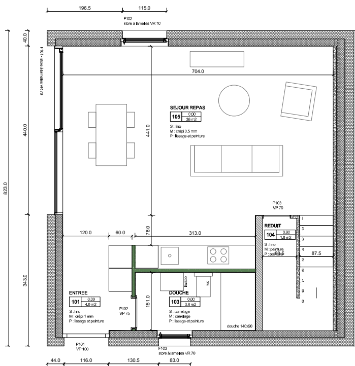
plan rez _ 1:100
