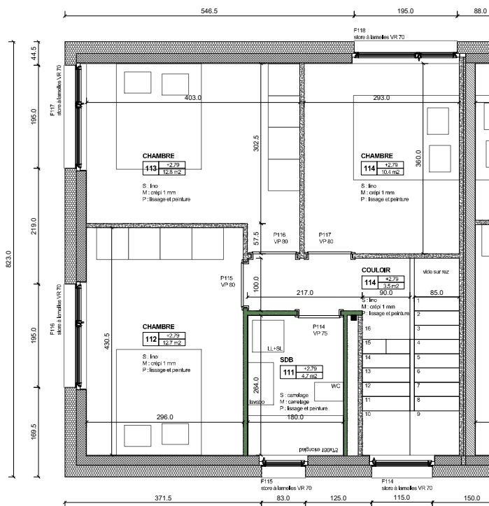
plan étage 1 _ 1:100
