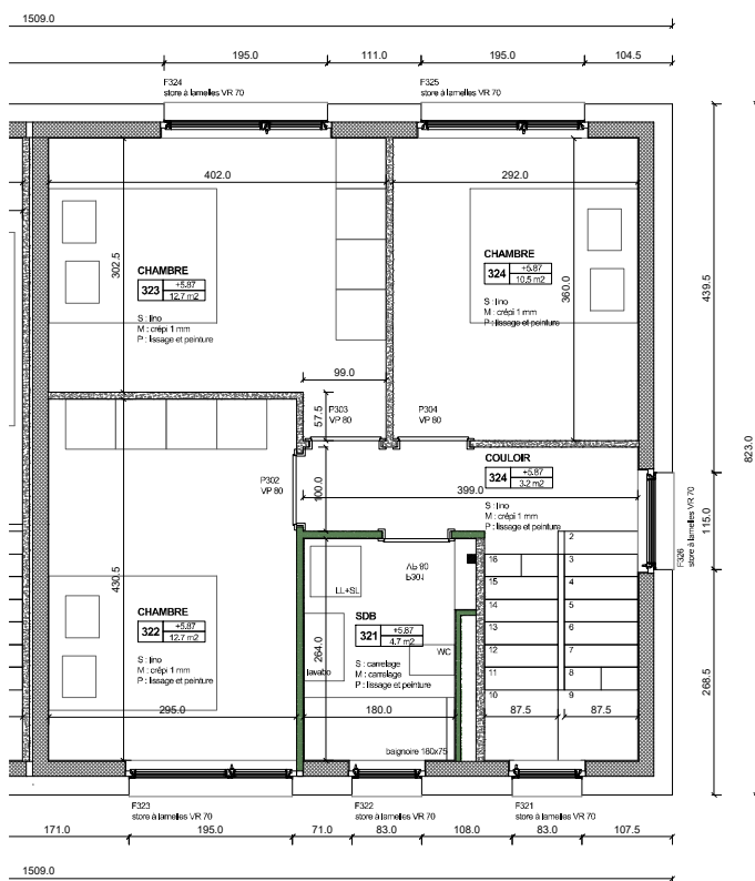
⌚ plan étage 2 _ 1:100
