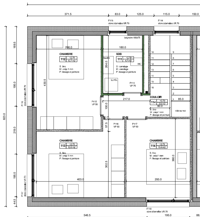
plan étage 1 _ 1:100
