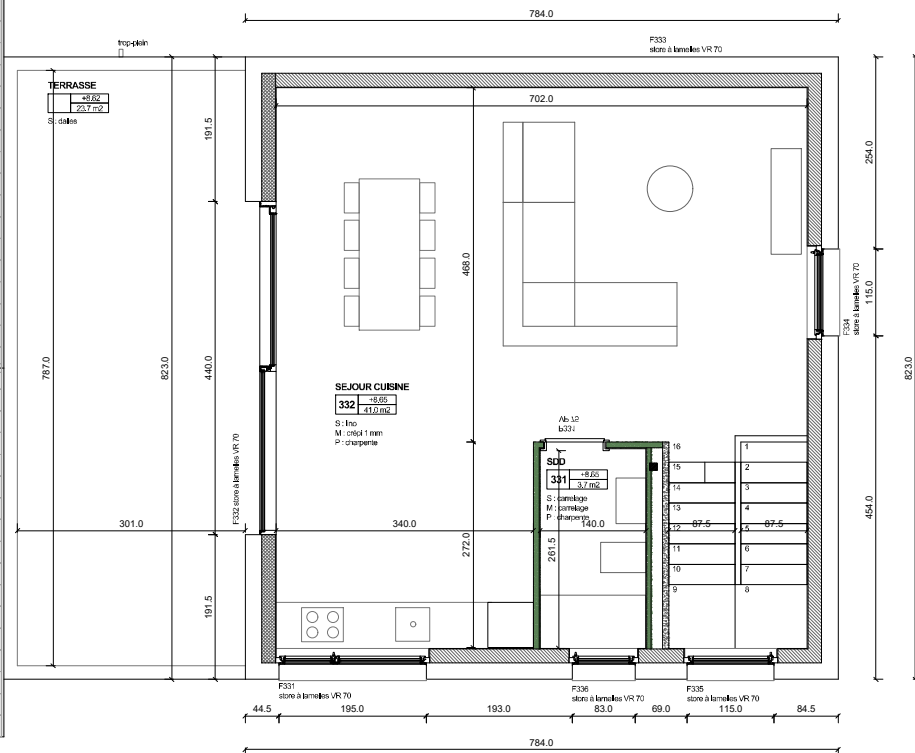
Surface villa (Sbp) : 130 m2 Surface terrasse : 24 m2 Parking : P2 (couvert) P14 (extérieur)
