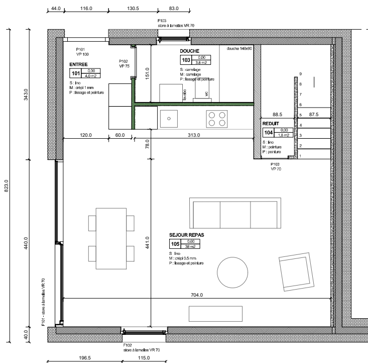
plan rez _ 1:100
