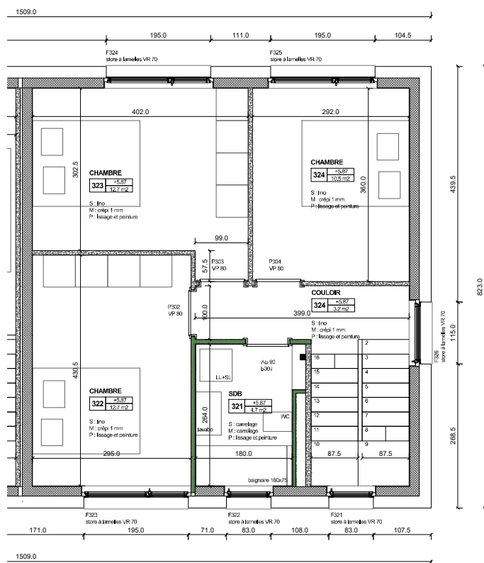
⌚ plan étage 2 _ 1:100
