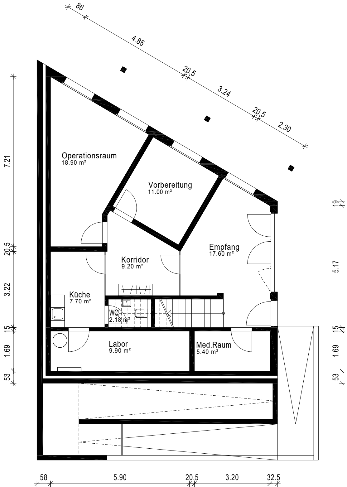
Untergeschoss
