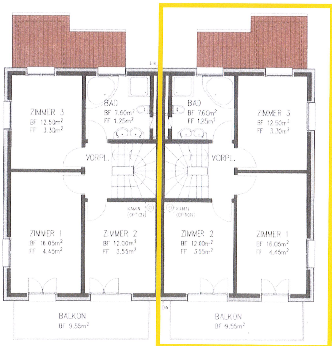
Obergeschoss 1:100
