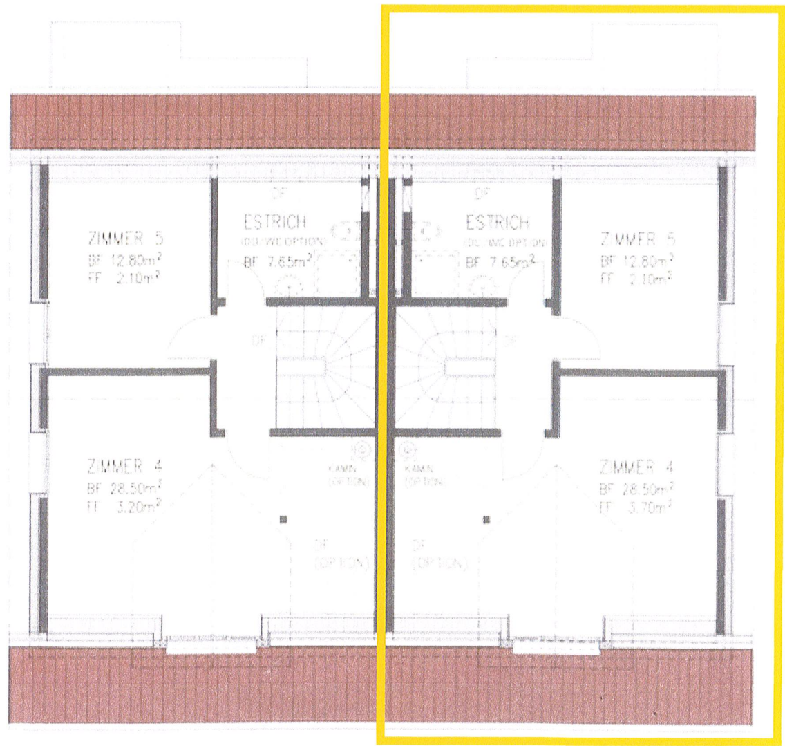
Dachgeschoss 1:100
