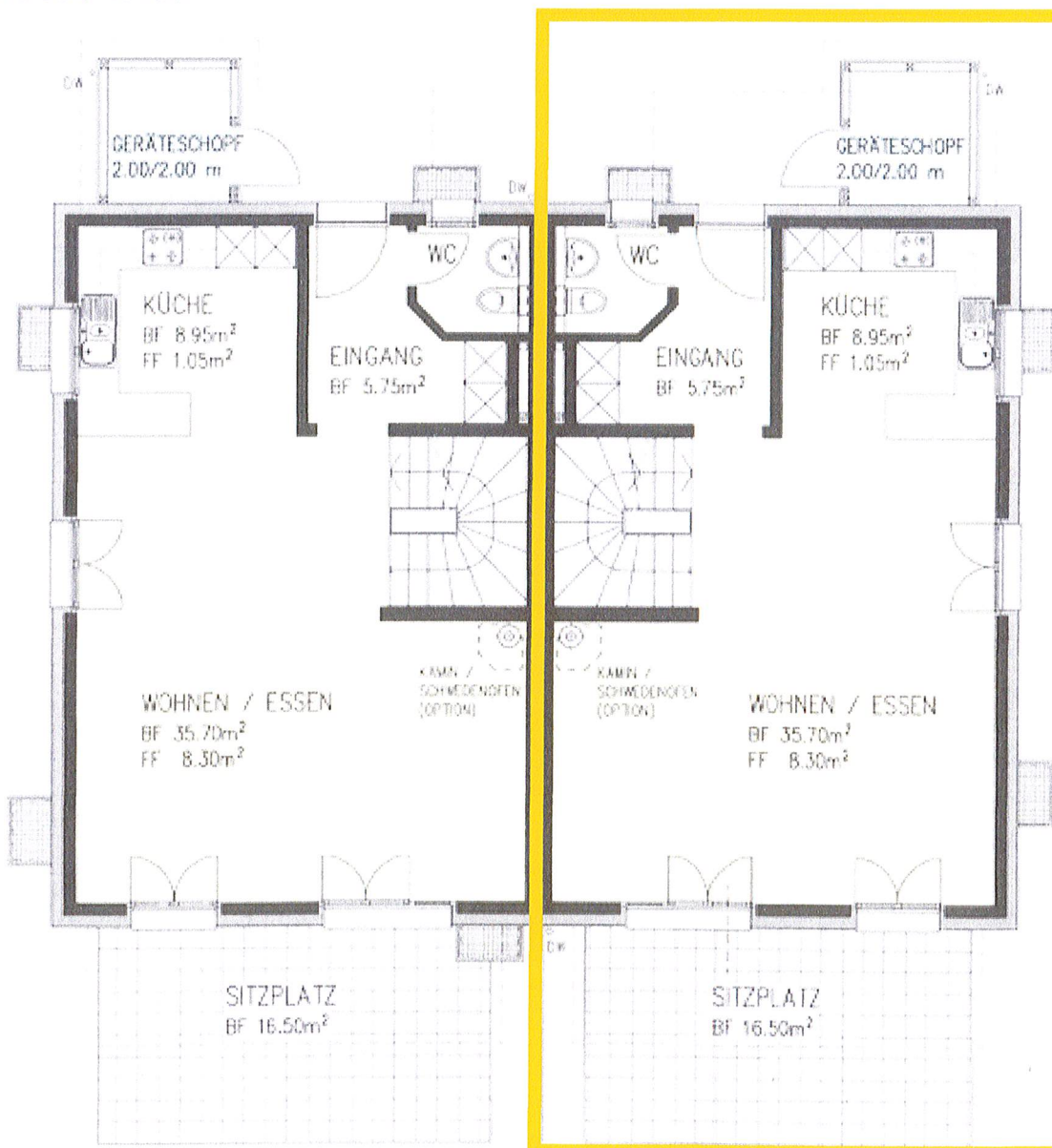
Erdgeschoss 1:100
