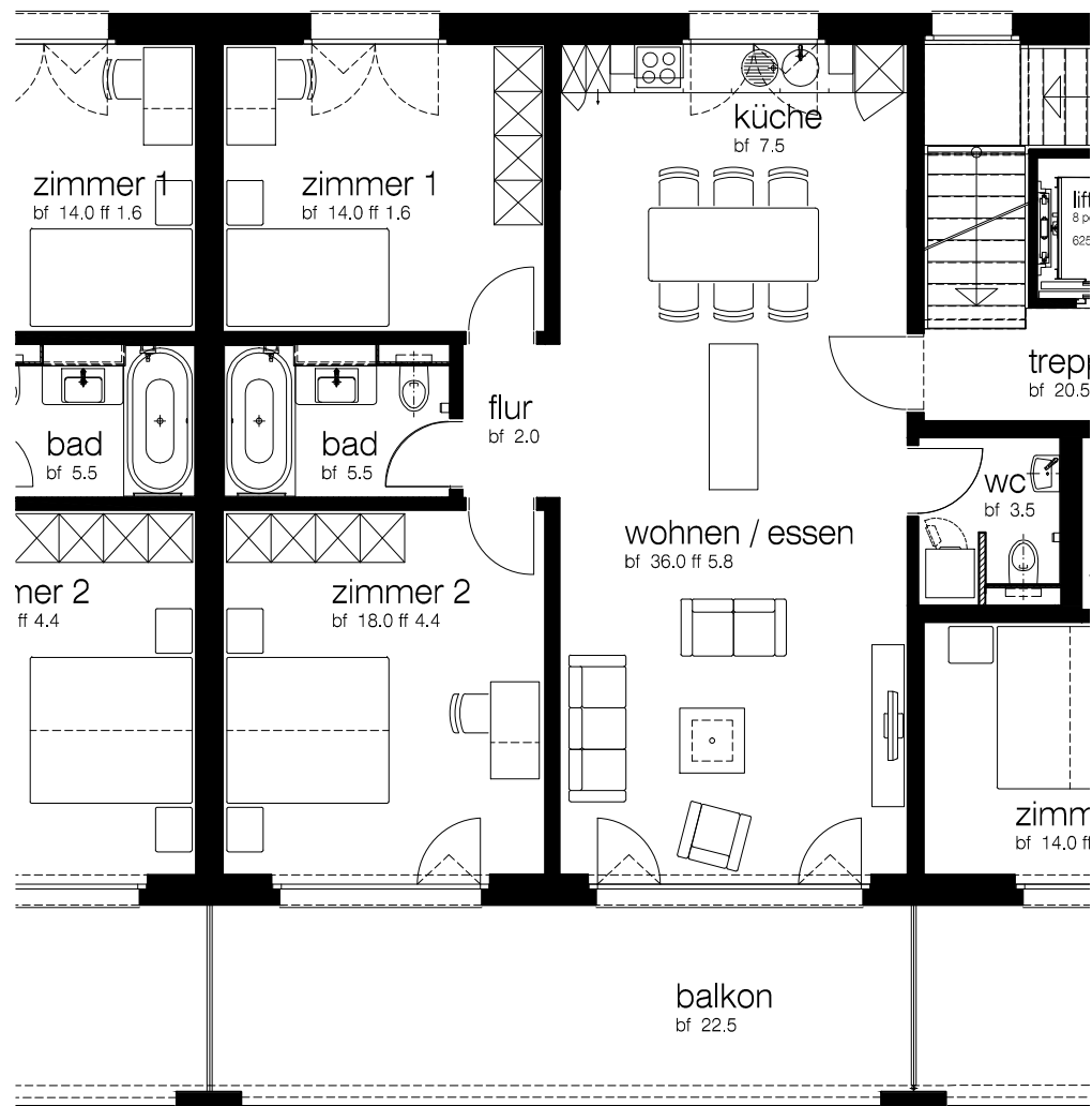
grundrissmasstab 1:100
