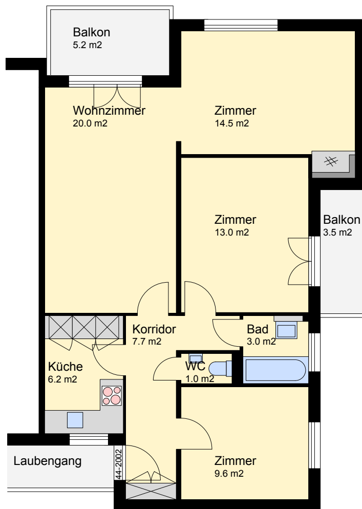
Willikonerstrasse 44, 8618 Oetwil am See 4 Zimmerwohnung 2. OG / Nr. 2002 Total 75.0 m 2 Grundrissplan Mst 1:100
