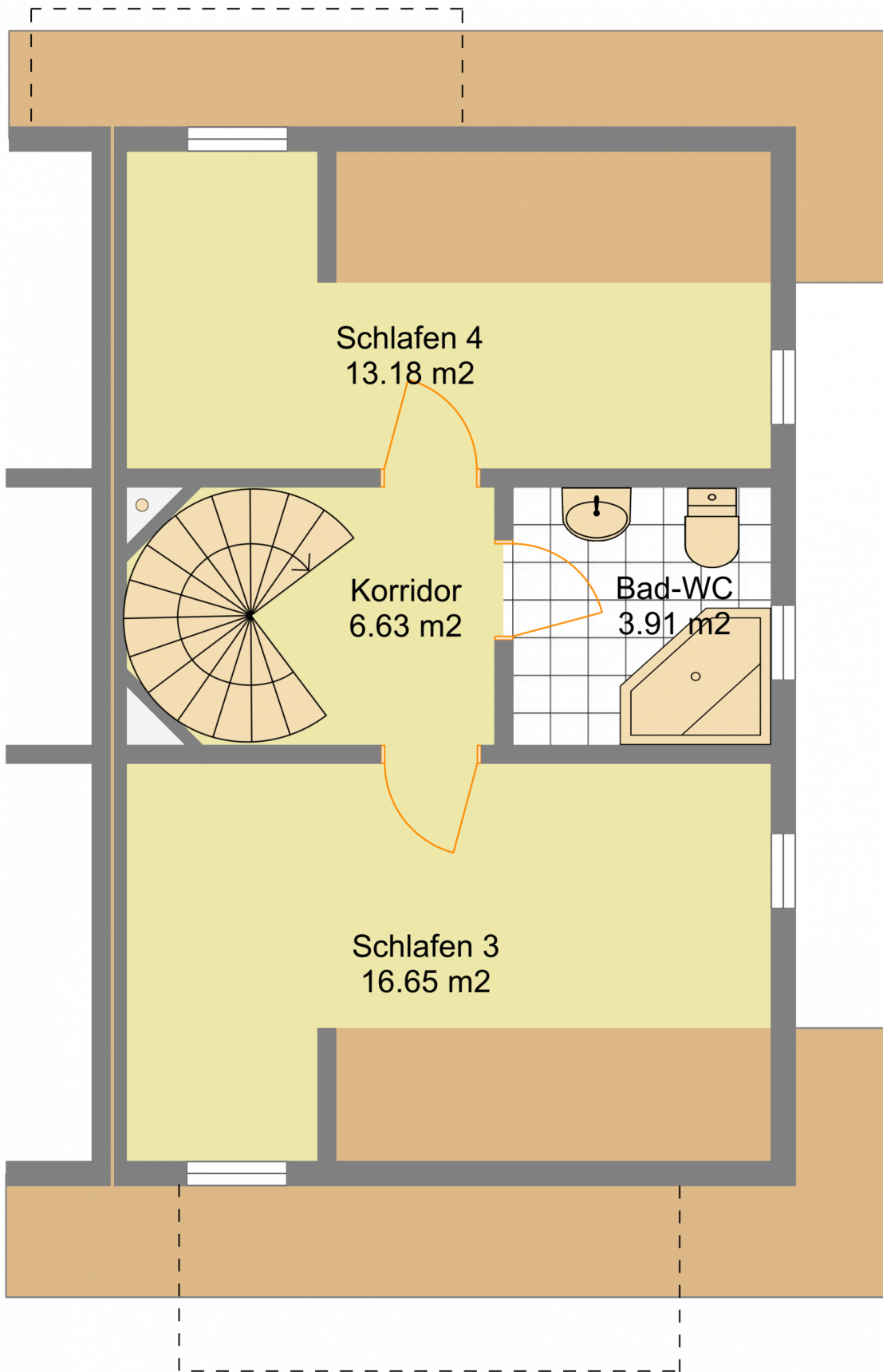
Dachgeschoss
