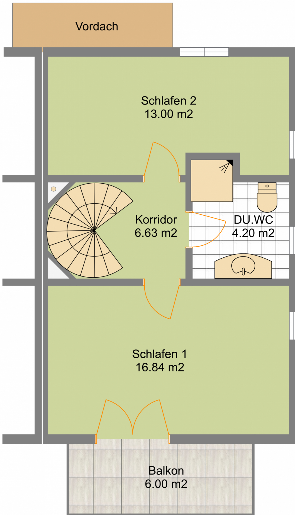
Obergeschoss
