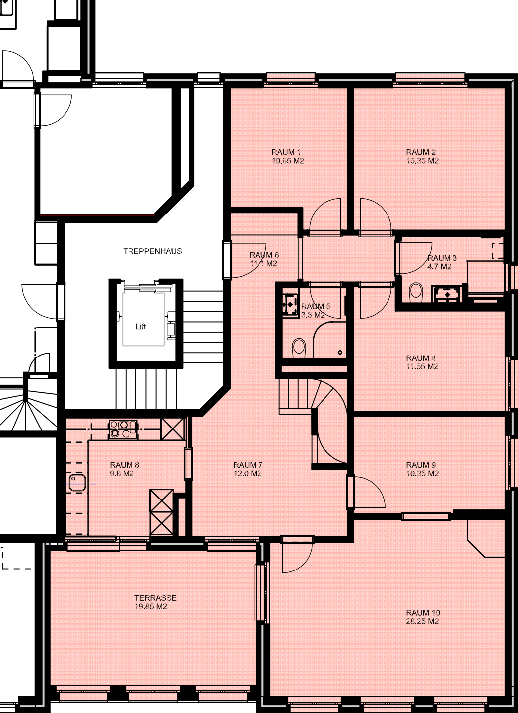
WOHNUNG 3. OBERGESCHOSS
