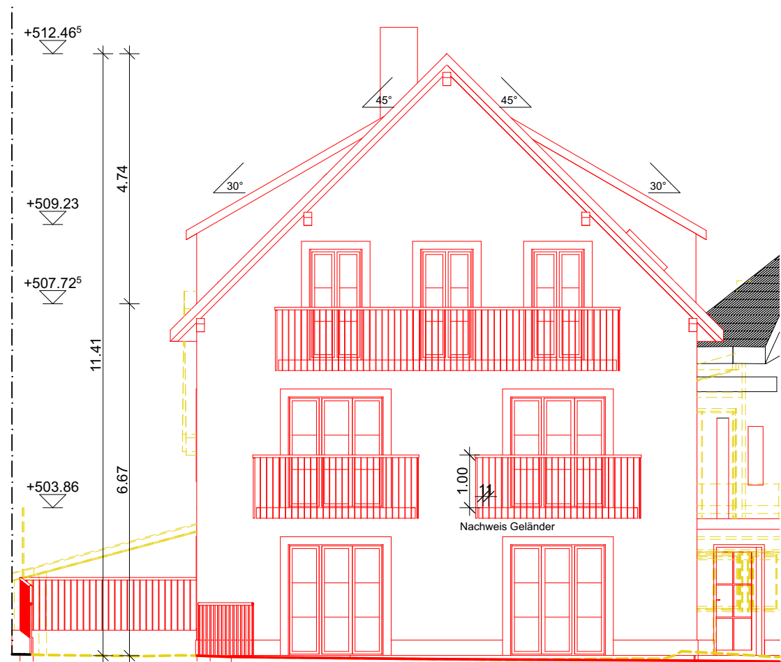
Südfassade
