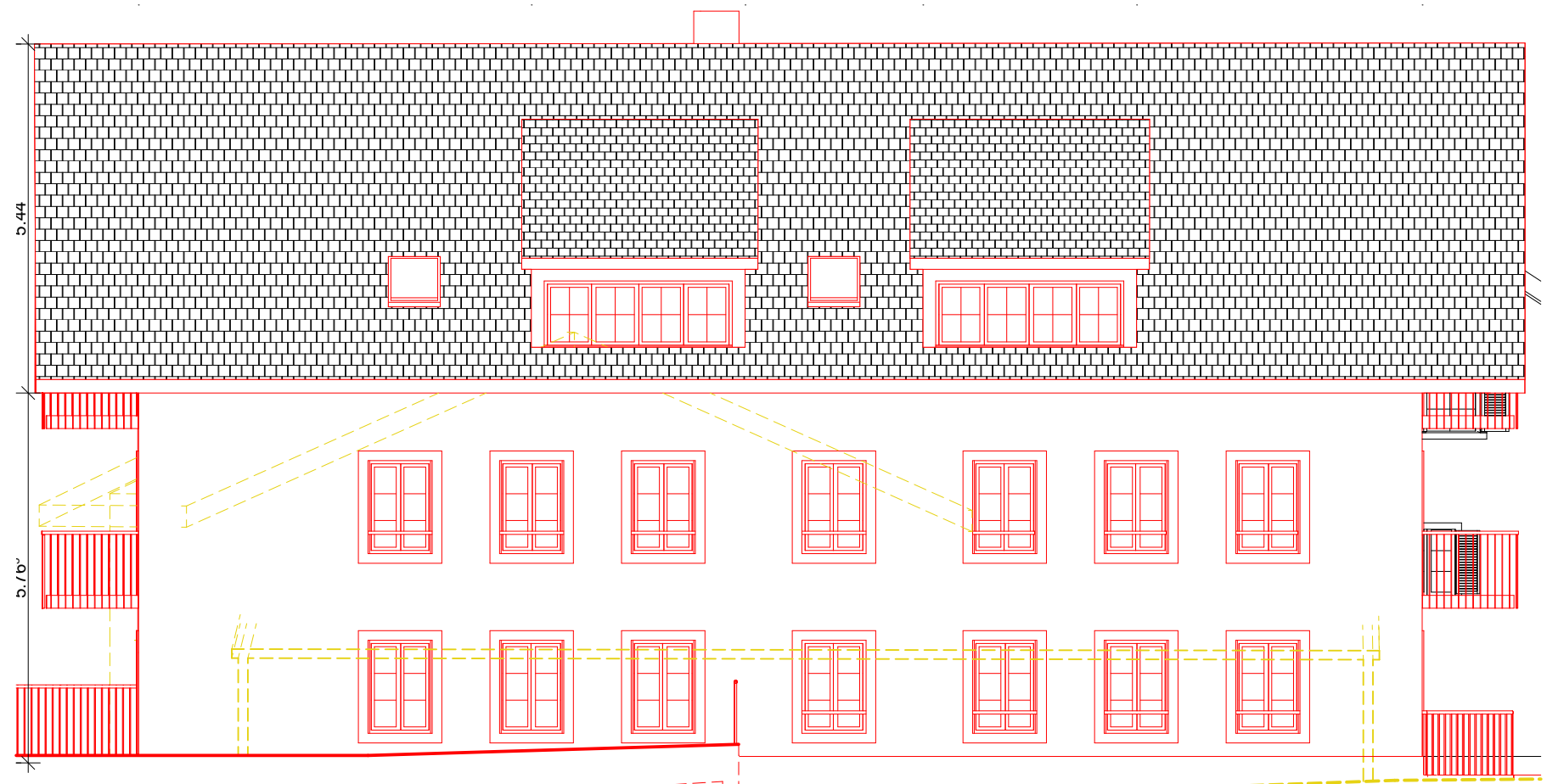
Westfassade
