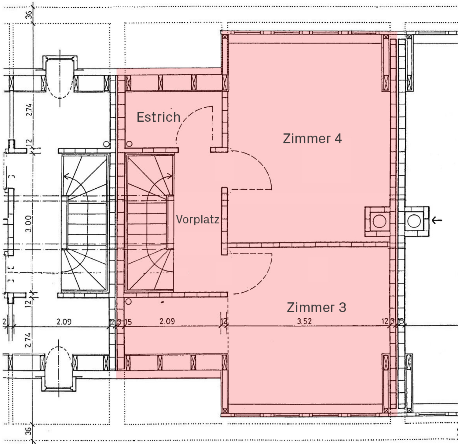
Dachgeschoss
