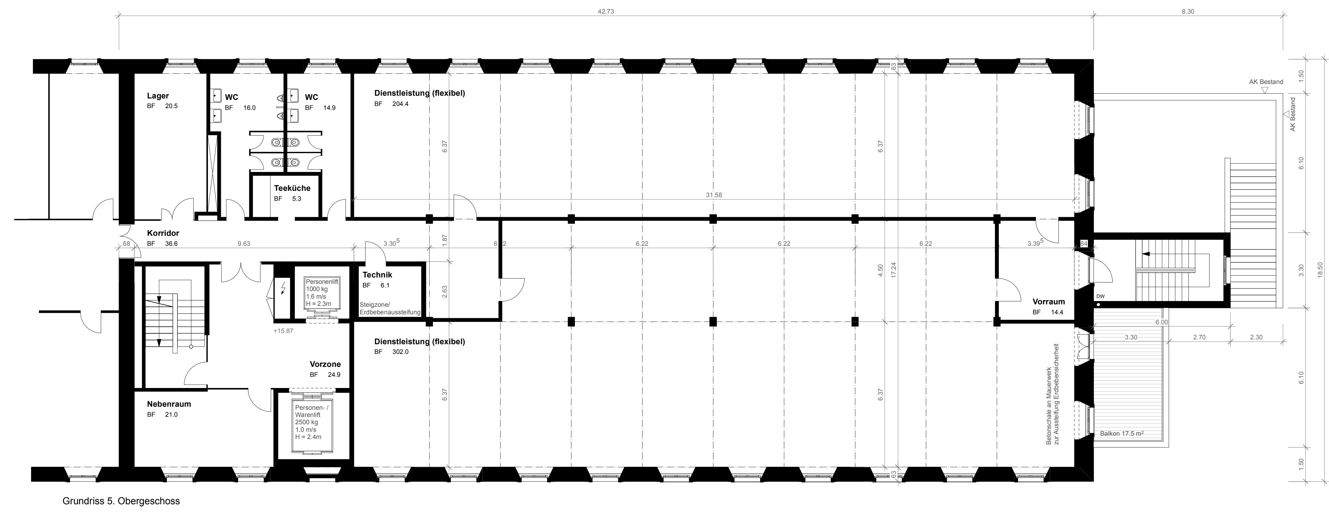
Grundriss 5. Obergeschoss
