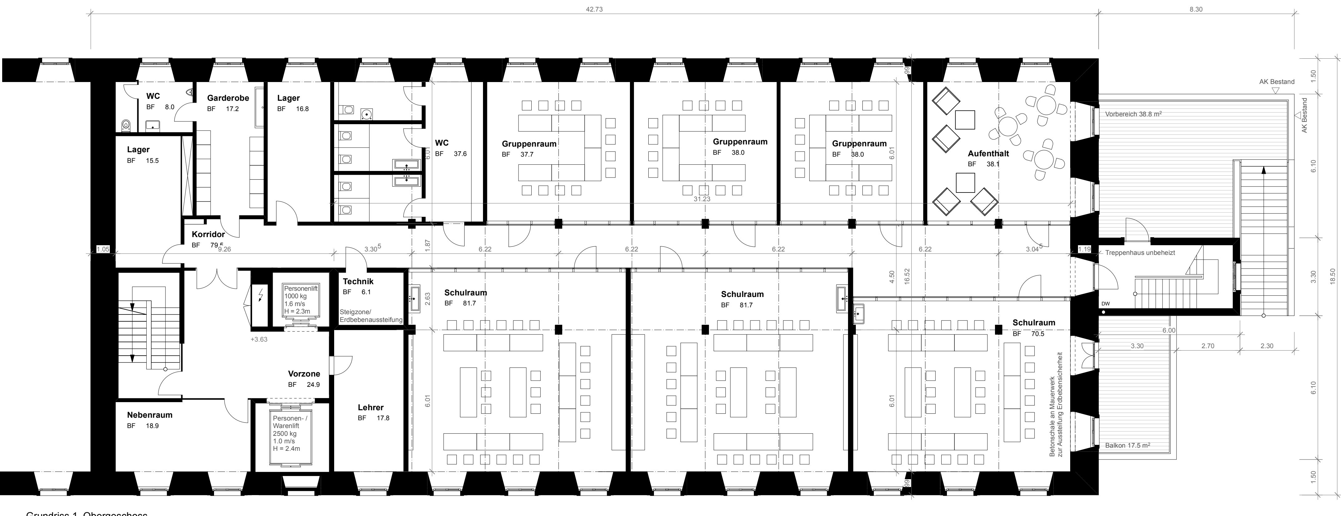
Grundriss 1. Obergeschoss
