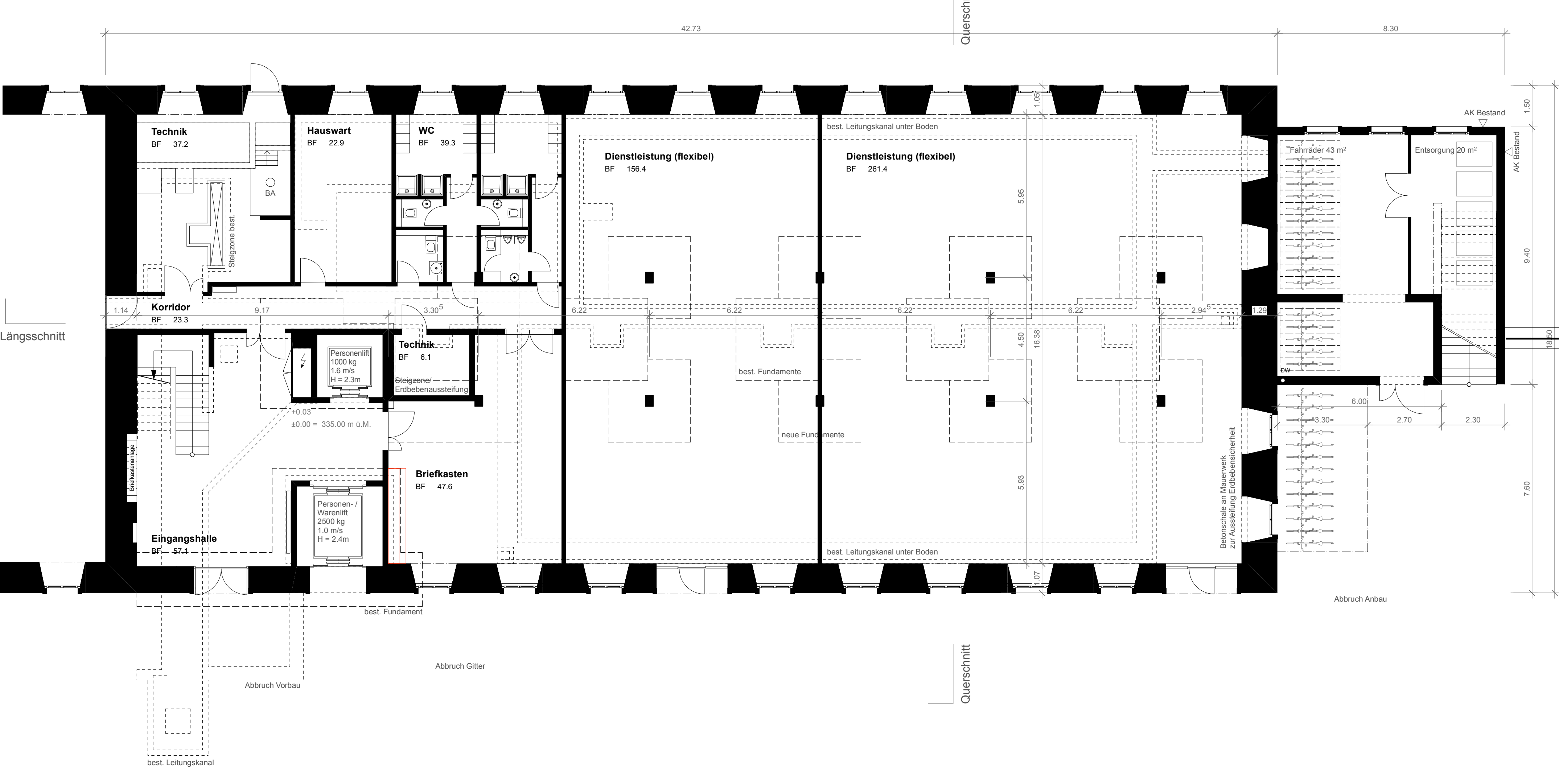
Grundriss Erdgeschoss
