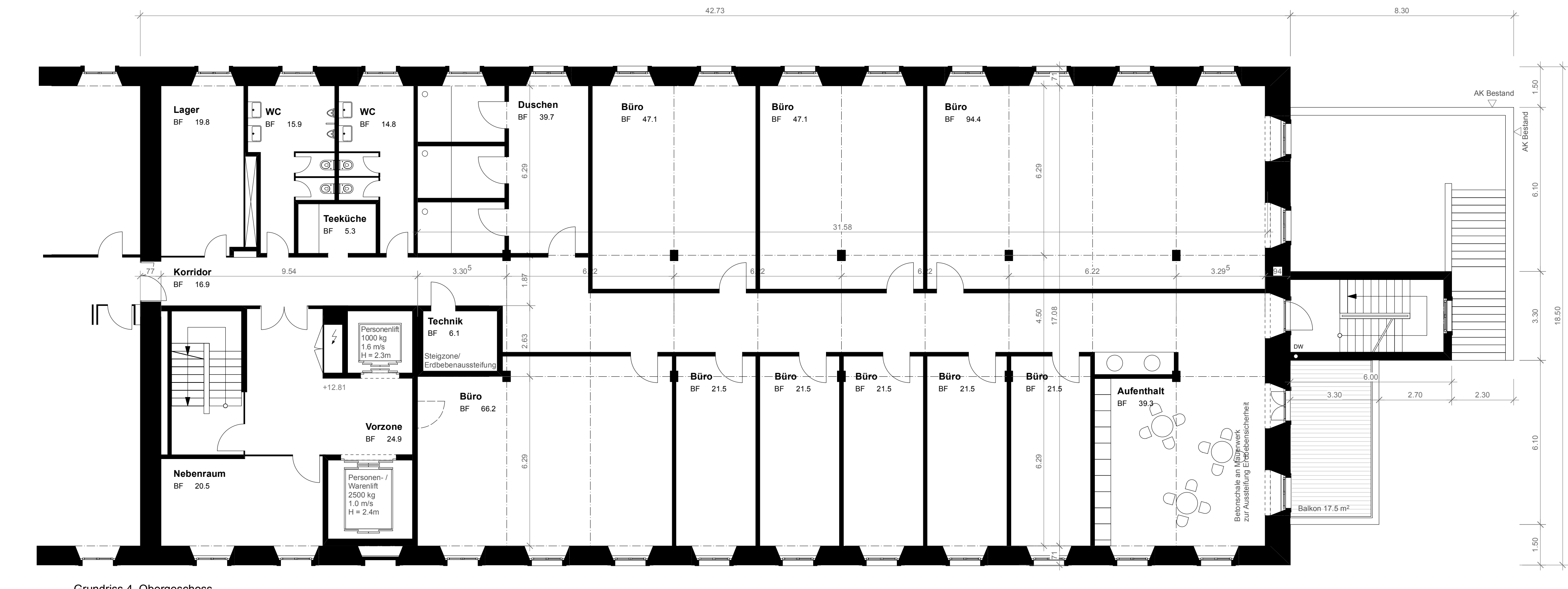
Grundriss 4. Obergeschoss
