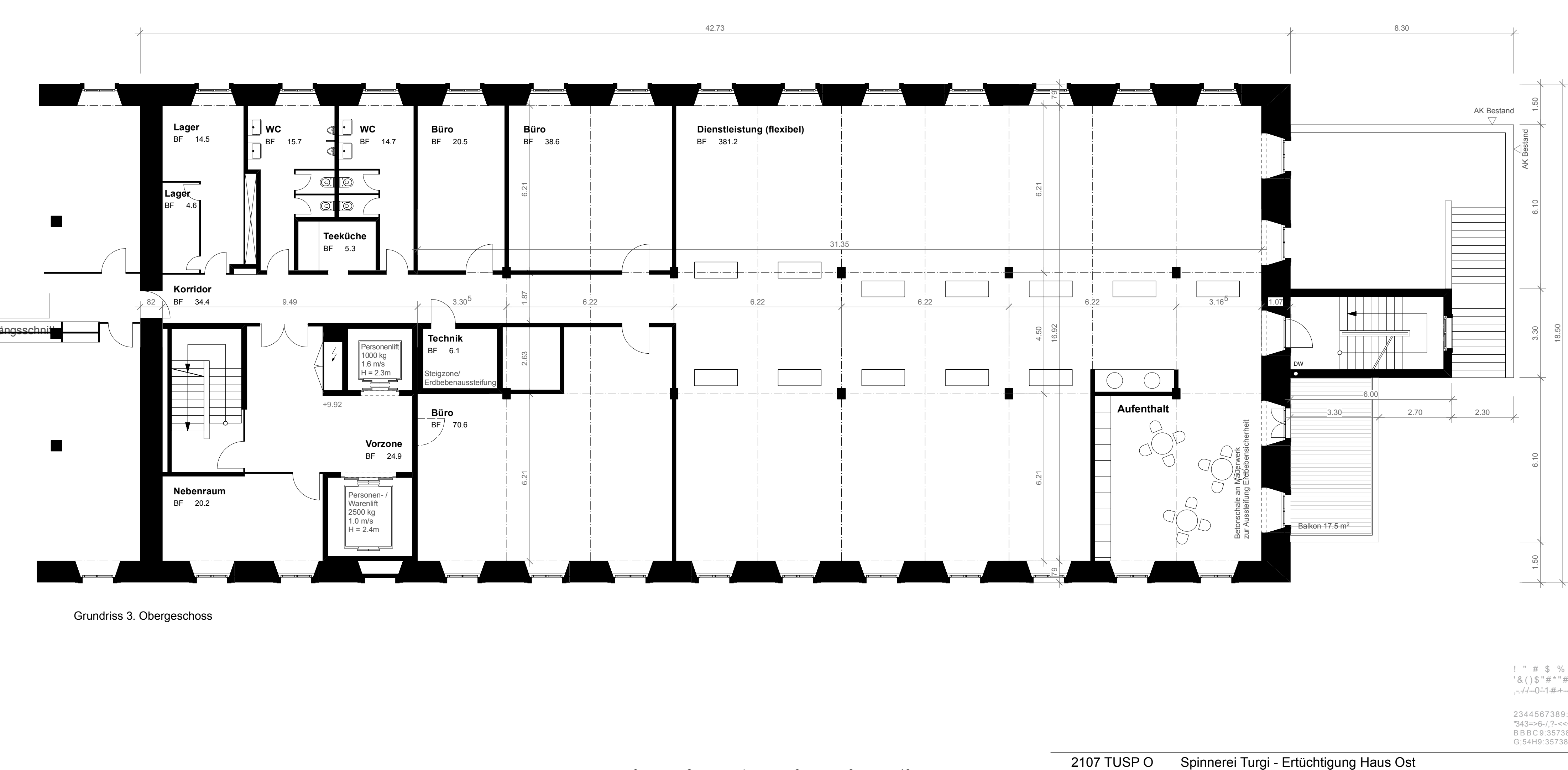
Grundriss 3. Obergeschoss
