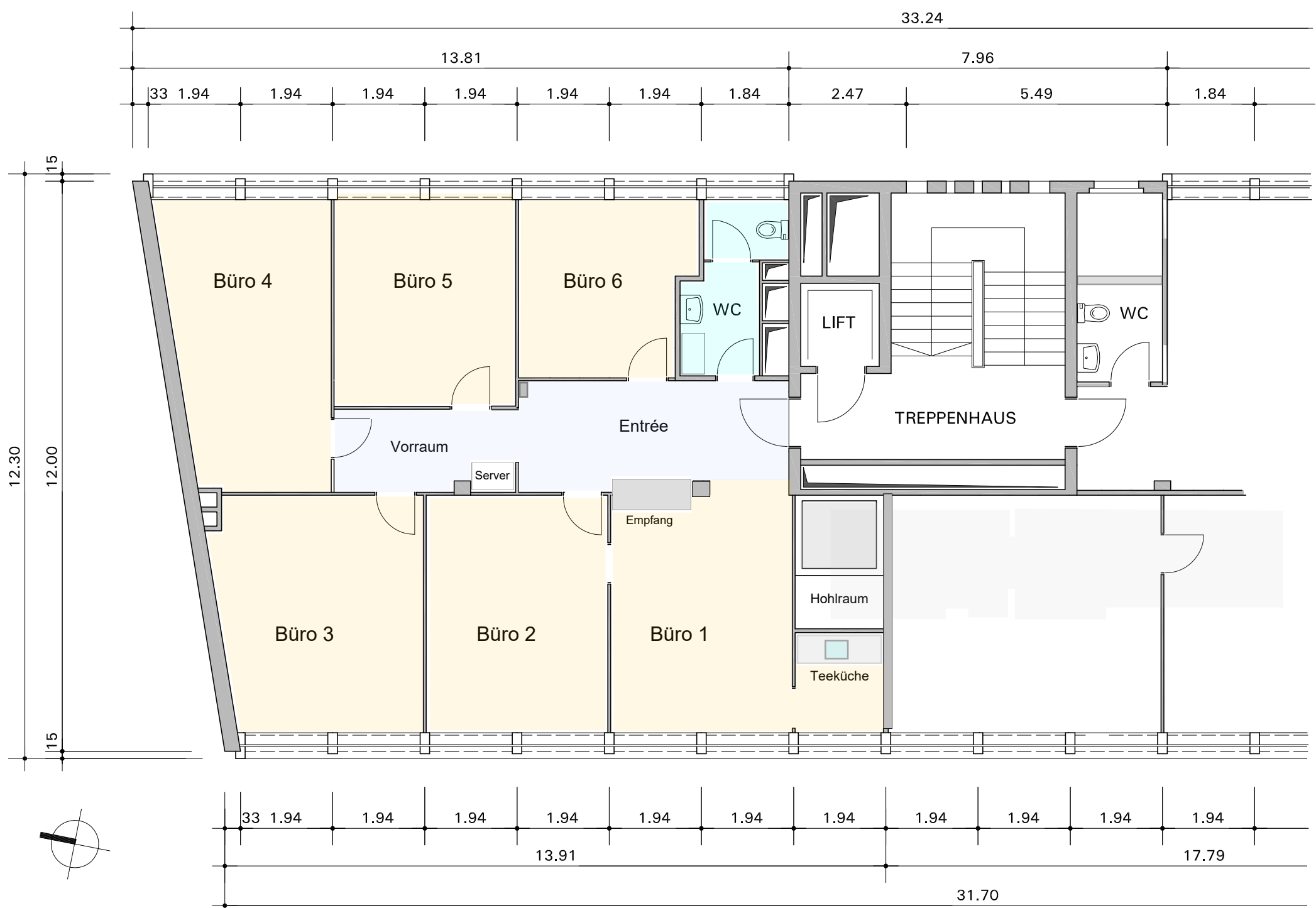
3. Obergeschoss (Nord) 1 : 100
