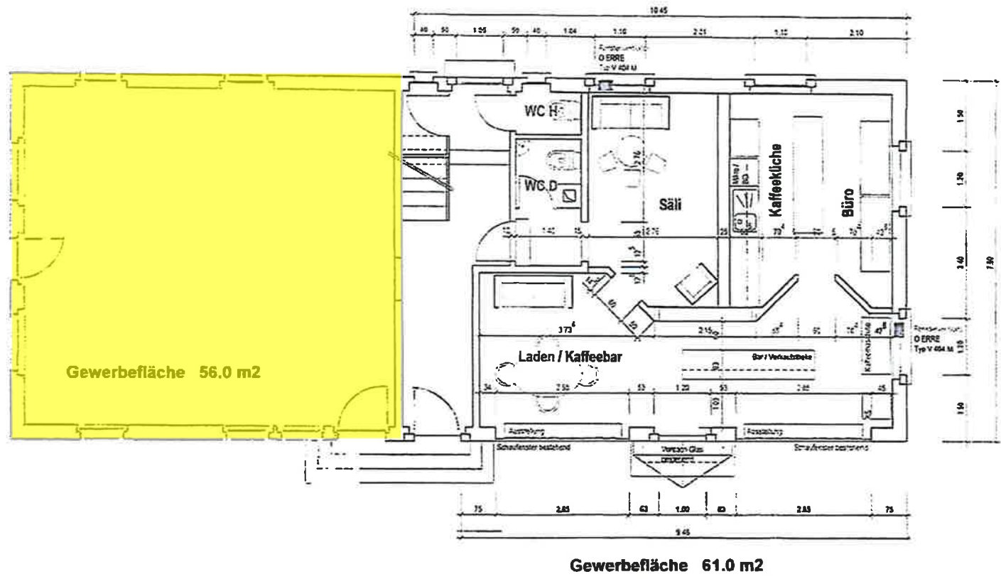
GUNDRISS ERDGESCHOSS, MST. 1:100
