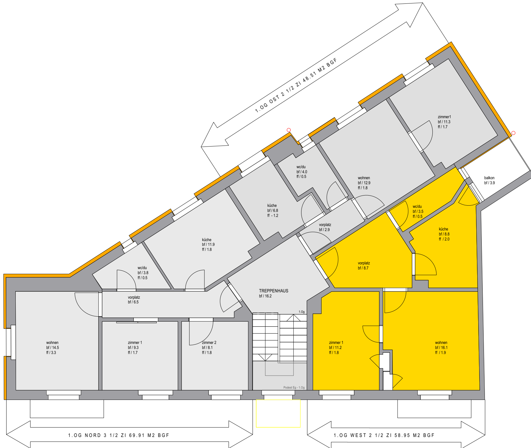
GRUNDRISSE 1:100
