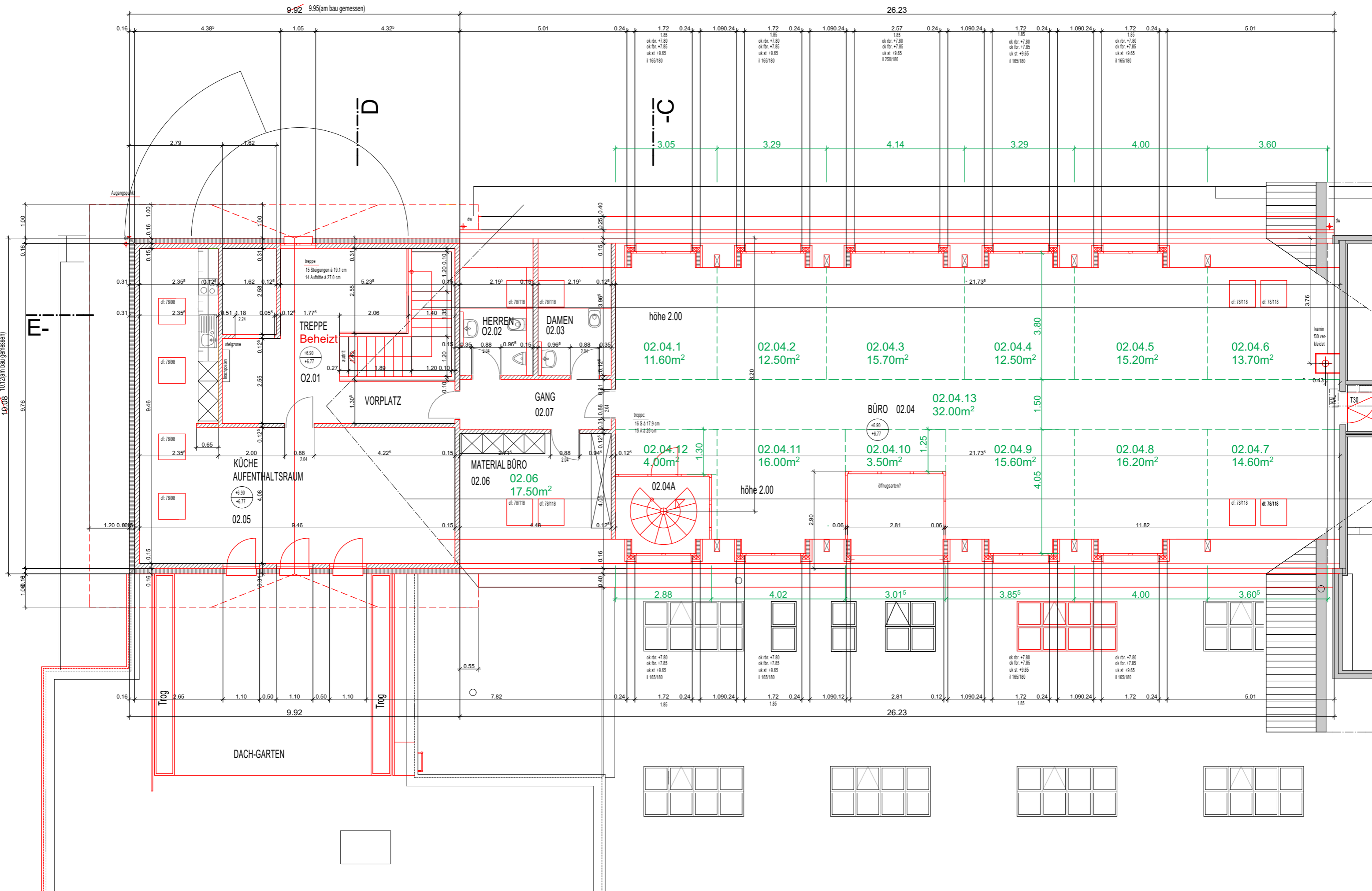
2. Obergeschoss Mst. 1:100
