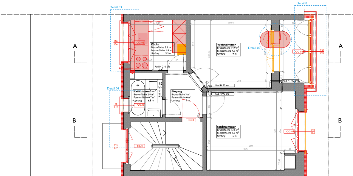
Obergeschoss x2
