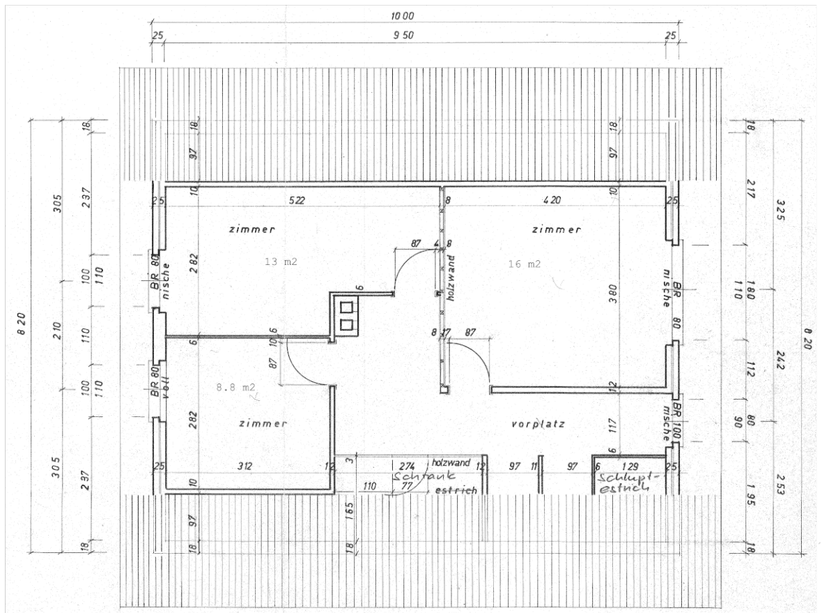
Obergeschoss 1:100
