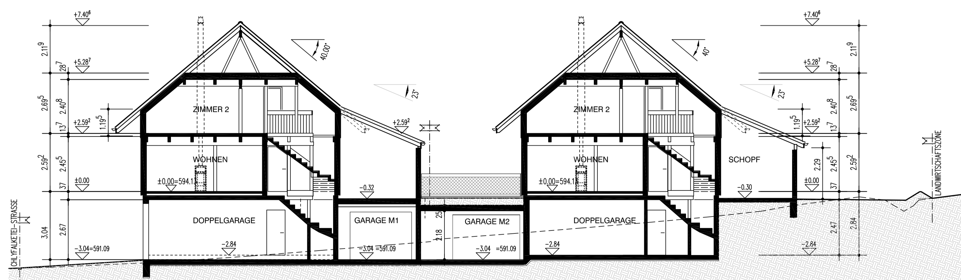
M1 SCHNITT
