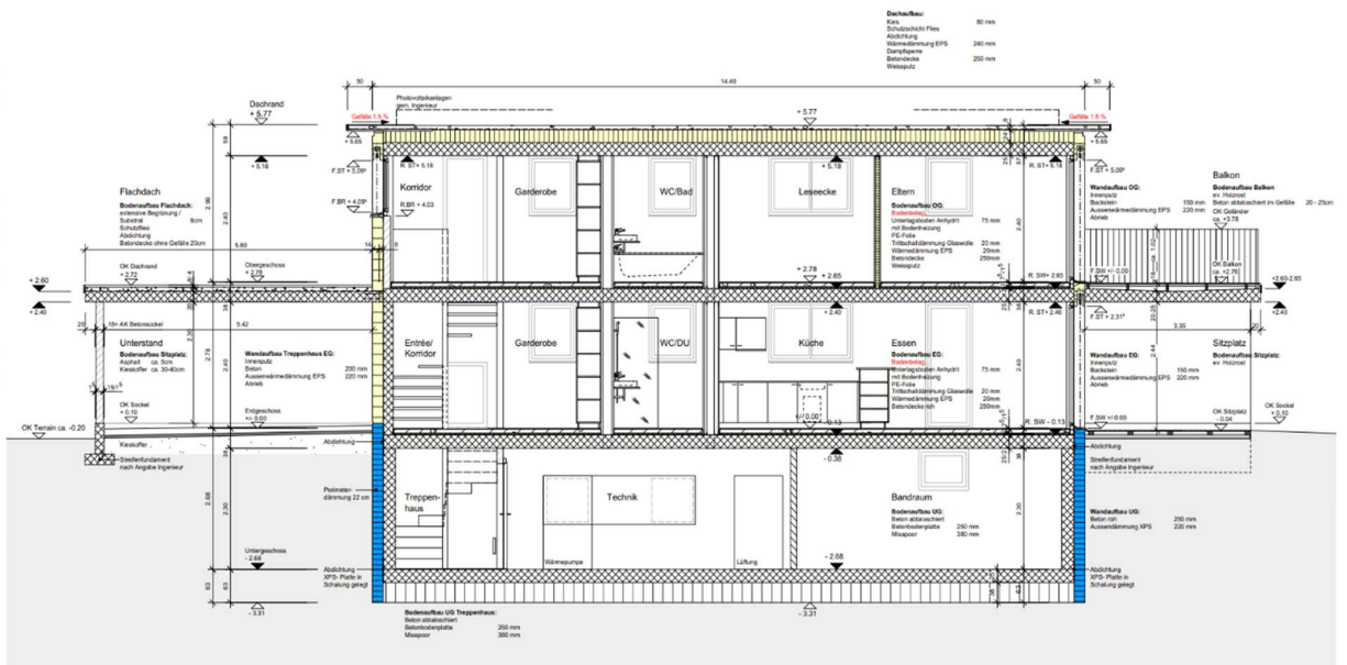
SCHNITT B-B
