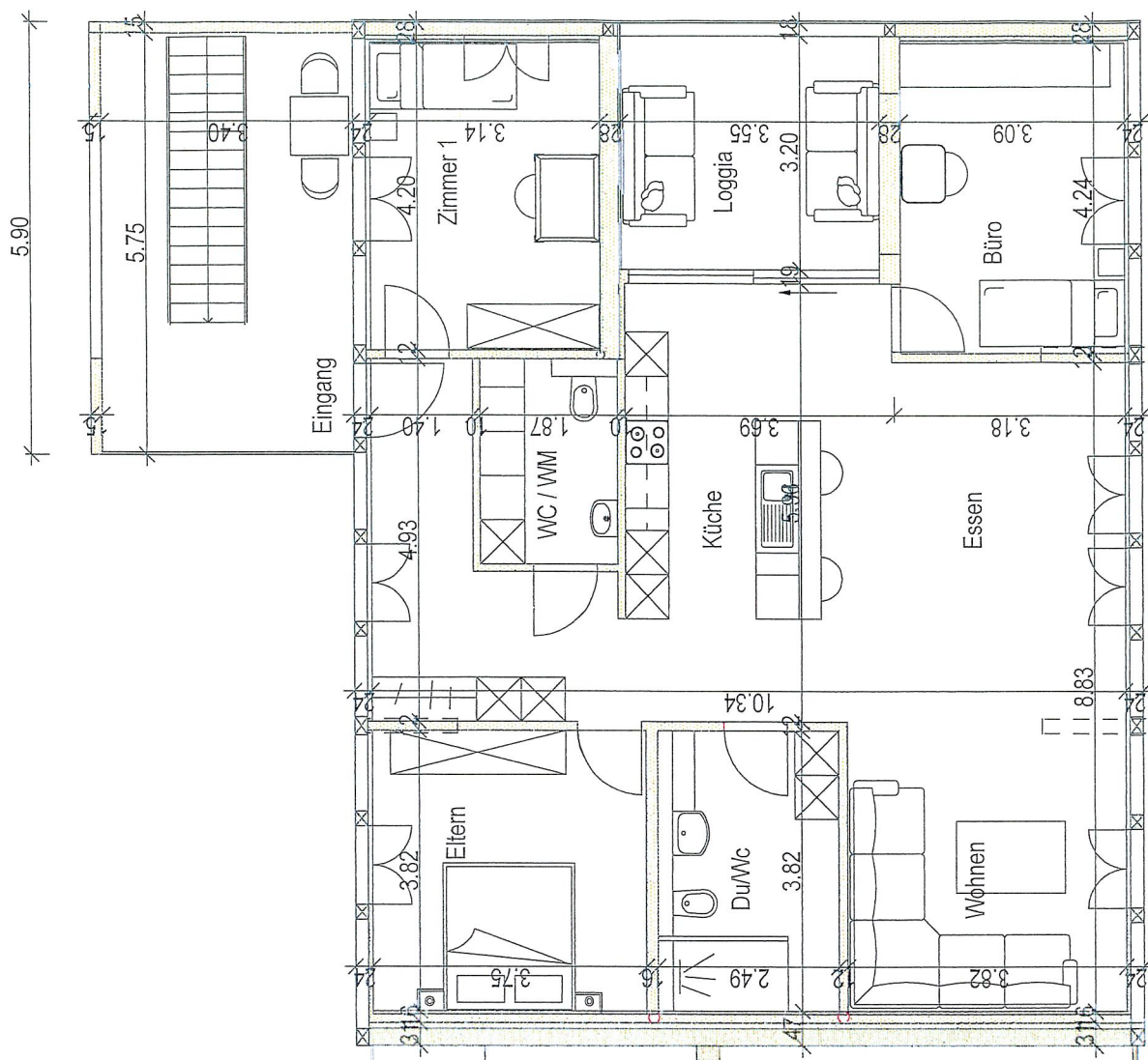
Grundriss OG Stallteil
