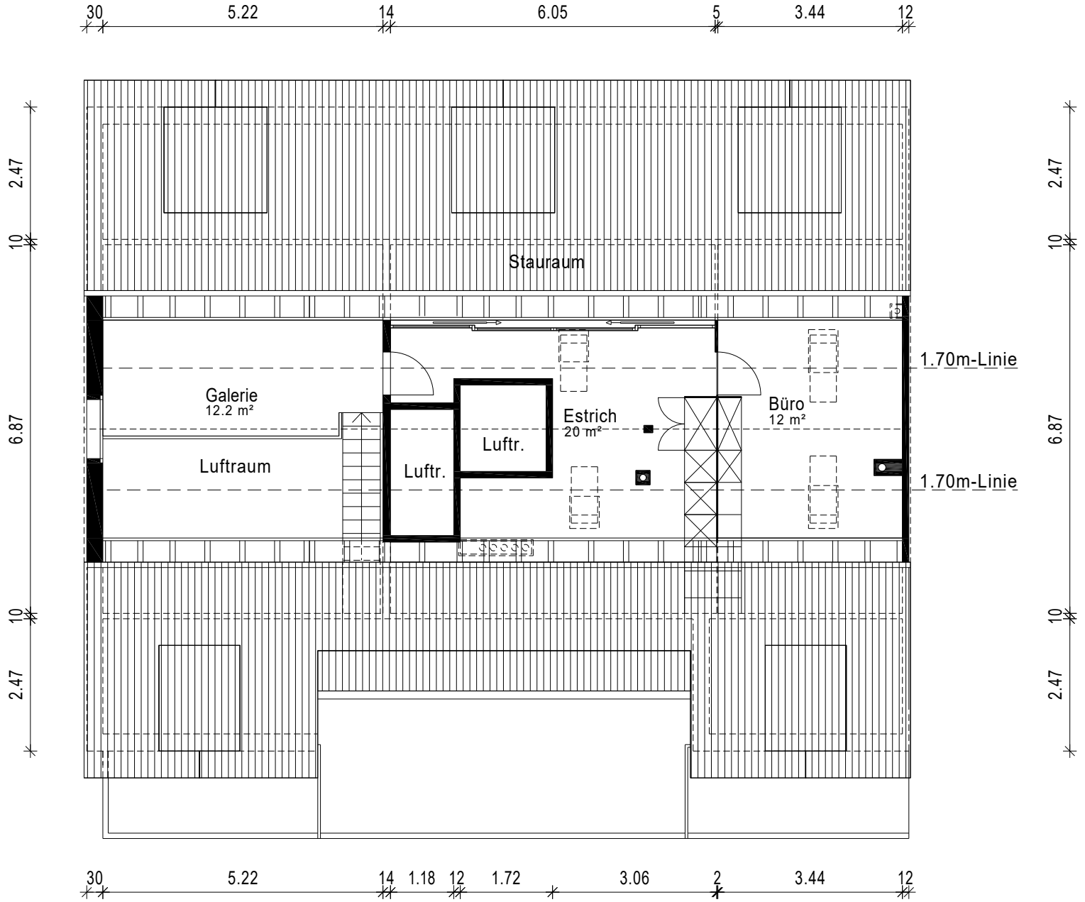
Galeriegeschoss
