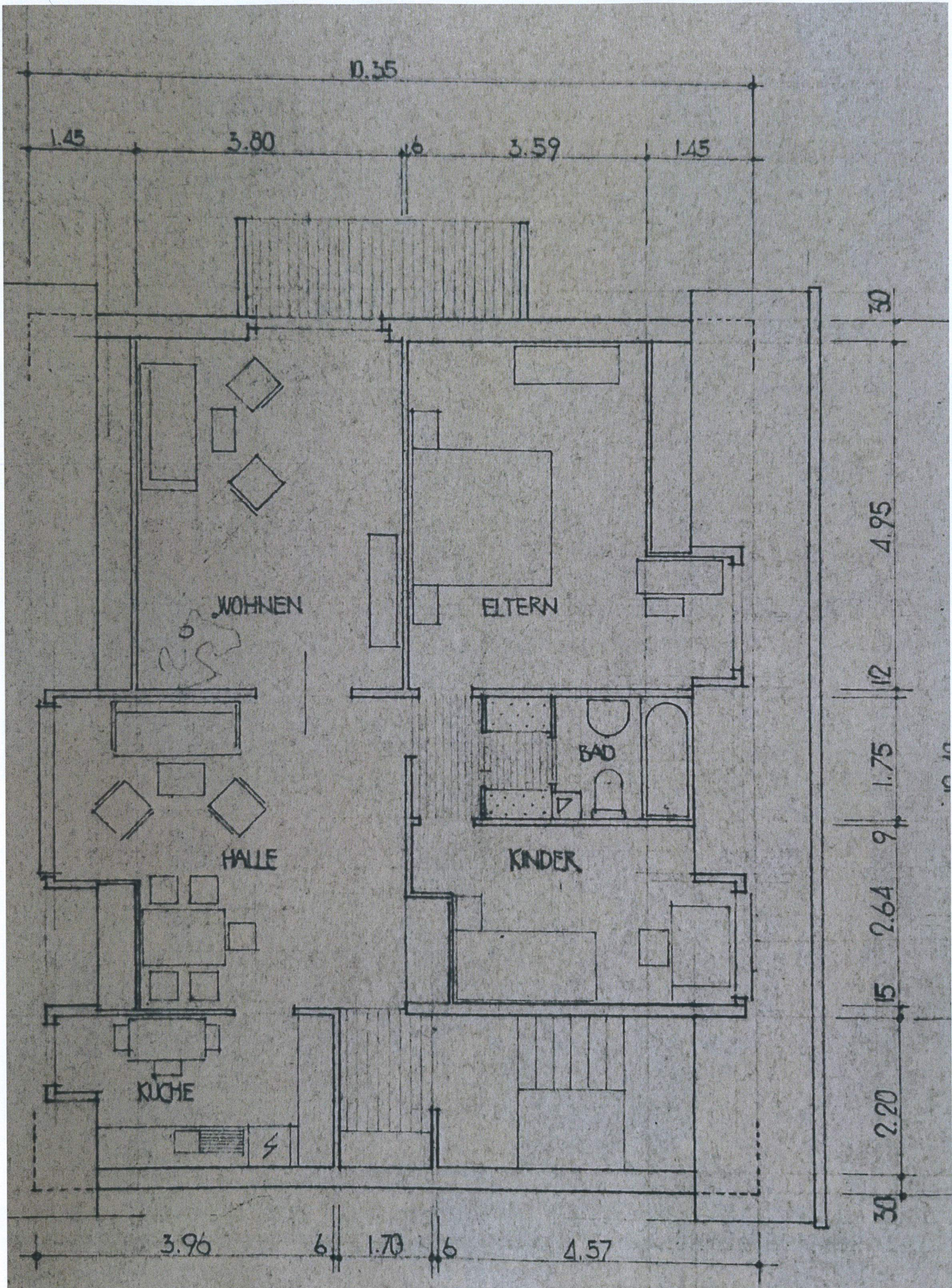
GRUNDRISS DACHSTOCK
